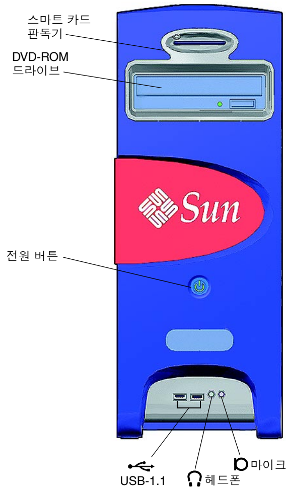
그림 1-3 전면 패널 구성
