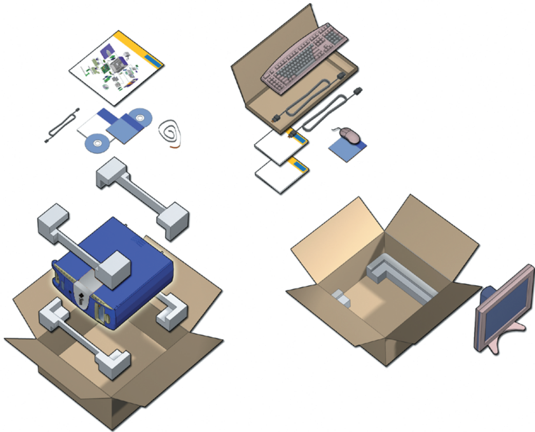
ABBILDUNG 1-2 Auspacken der Workstation
