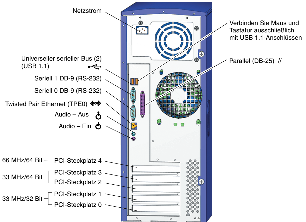
ABBILDUNG 1-4 Übersicht über die Rückseite
