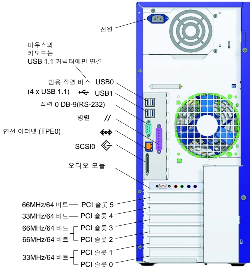
그림 1-4 후면 패널 구성
