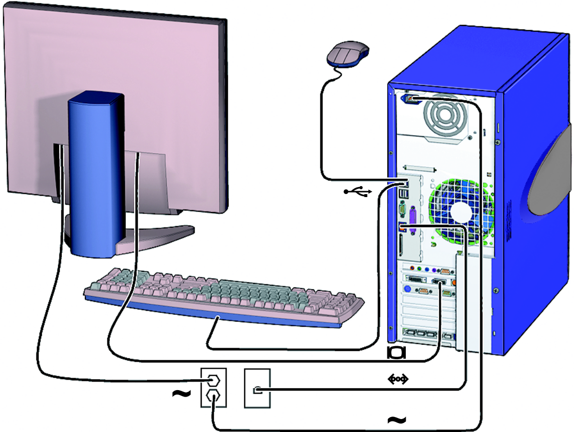
그림 1-6 Sun Blade 2500 워크스테이션 케이블 연결
