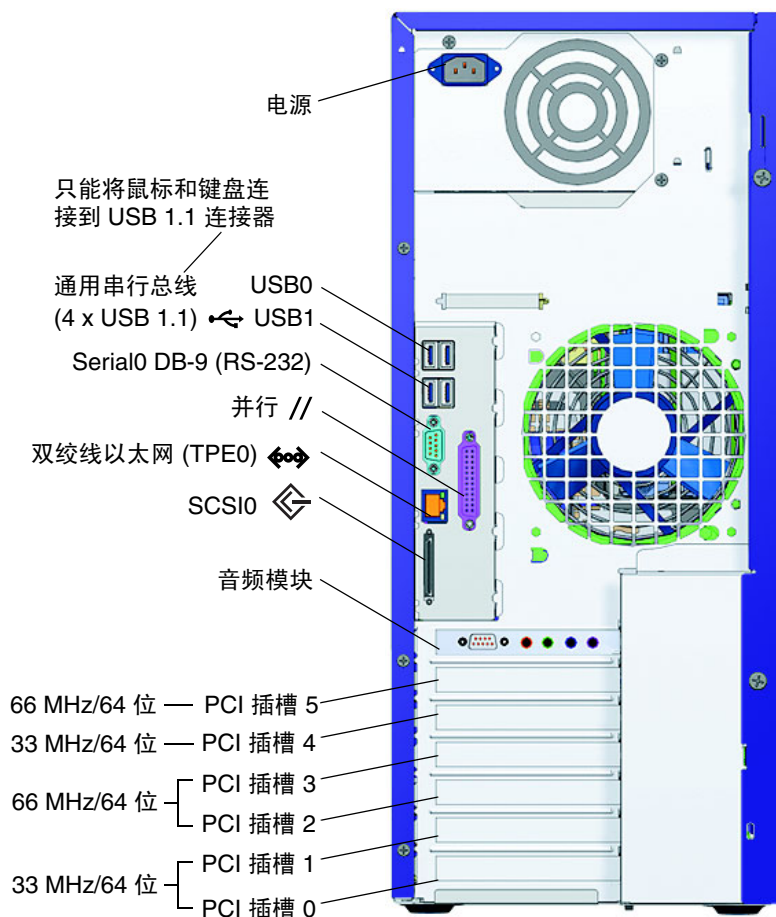
图 1-4 后面板视图
