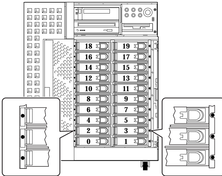
FIGURA 3-2 Números de las ranuras de disco y ubicación de los LED
