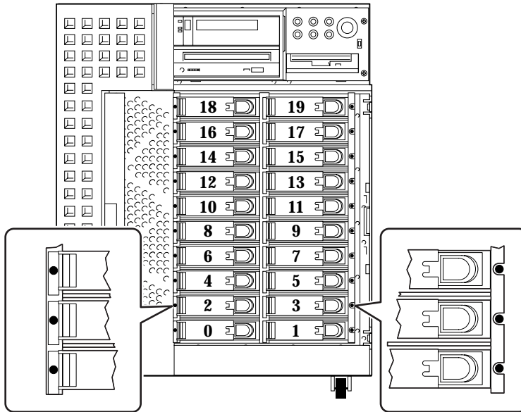
FIGURA 3-3 Números de las ranuras de discos y ubicación de los LED
