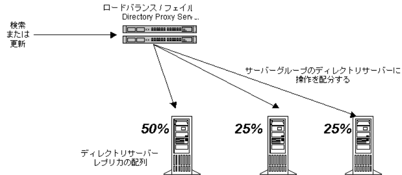
図 8-2 複数の LDAP ディレクトリレプリカ間でのロードバランス
