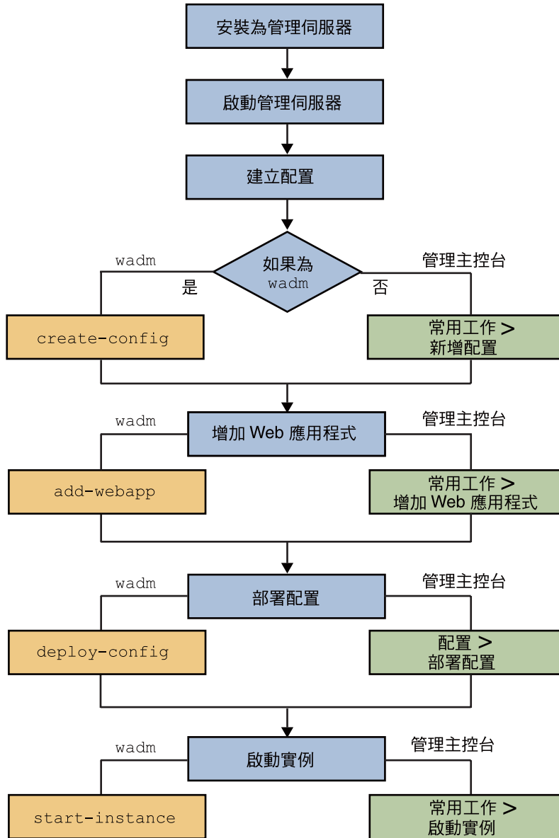
圖 4-1 說明在單一節點上部署 Web 伺服器的流程圖
