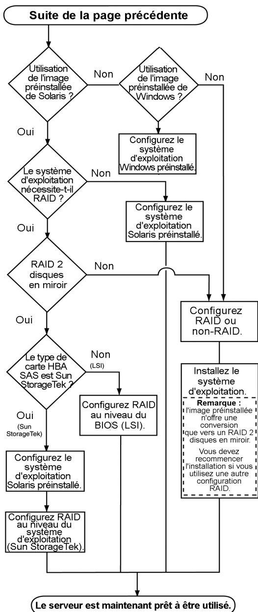
FIGURE 1-2 Procédure d'installation du serveur Sun Fire X4450 (Partie 2)
