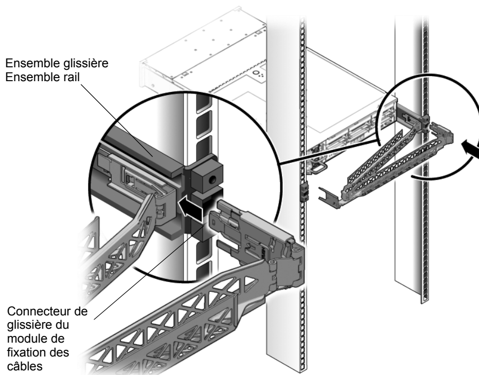
FIGURE 2-10 Insertion du connecteur de glissière du module de fixation des câbles à l'arrière de l'ensemble glissière droit
