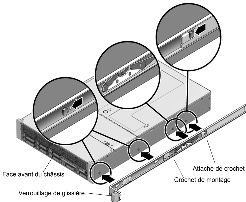
FIGURE 2-2 Alignement du crochet de montage sur le châssis du serveur
