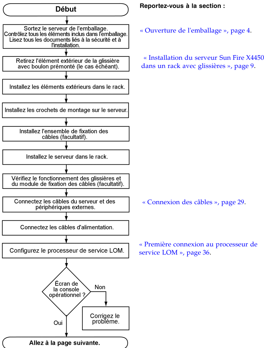
FIGURE 1-1 Procédure d'installation du serveur Sun Fire X4450 (Partie 1)
