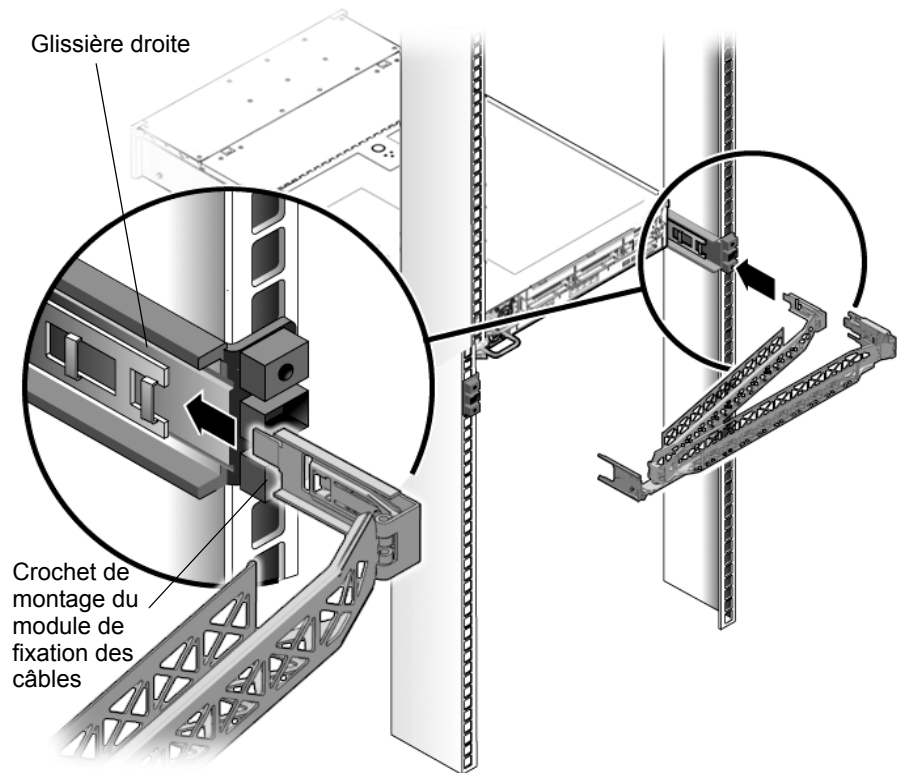
FIGURE 2-9 Insertion du crochet de montage du module de fixation des câbles à l'arrière de la glissière droite
