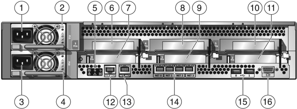
FIGURE 1-5 Panneau arrière
