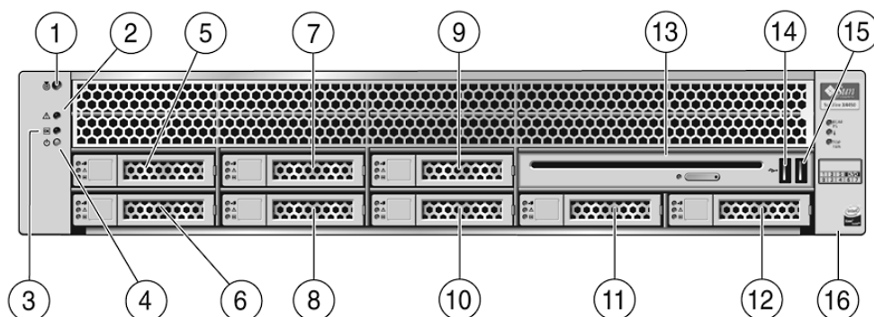
FIGURE 1-4 Panneau avant - illustration d'une configuration à 8 unités
