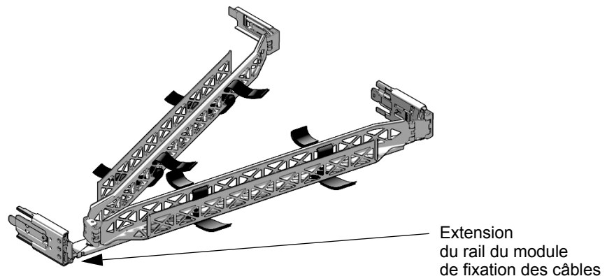
FIGURE 2-7 Module de fixation des câbles
