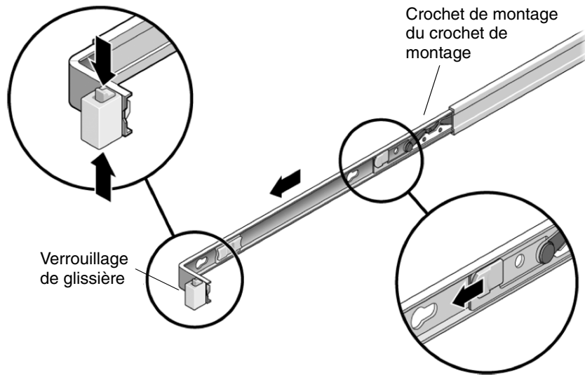
FIGURE 2-1 Désassemblage de la glissière avec boulon prémonté avant l'installation
