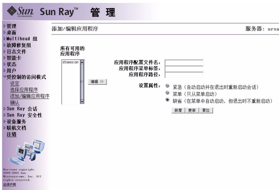
图 3 Sun Ray Server Software 的“添加/编辑应用程序”面板
