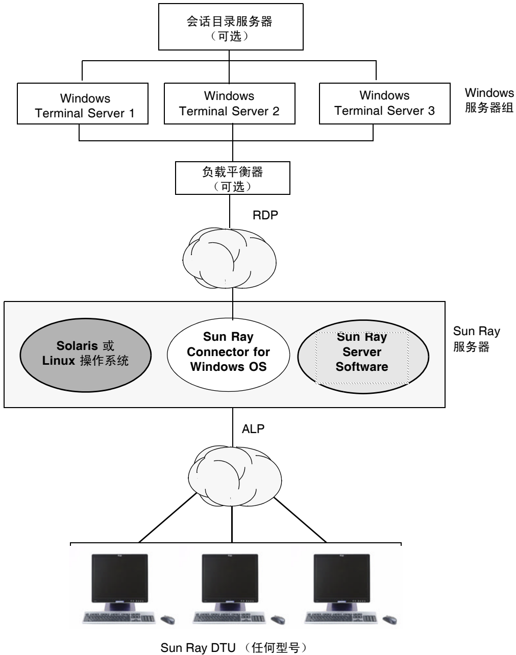
图 1 通过 RDP 和 ALP 协议建立的 Sun Ray-Windows 连接（其中负载均衡和会话目录为可选）
