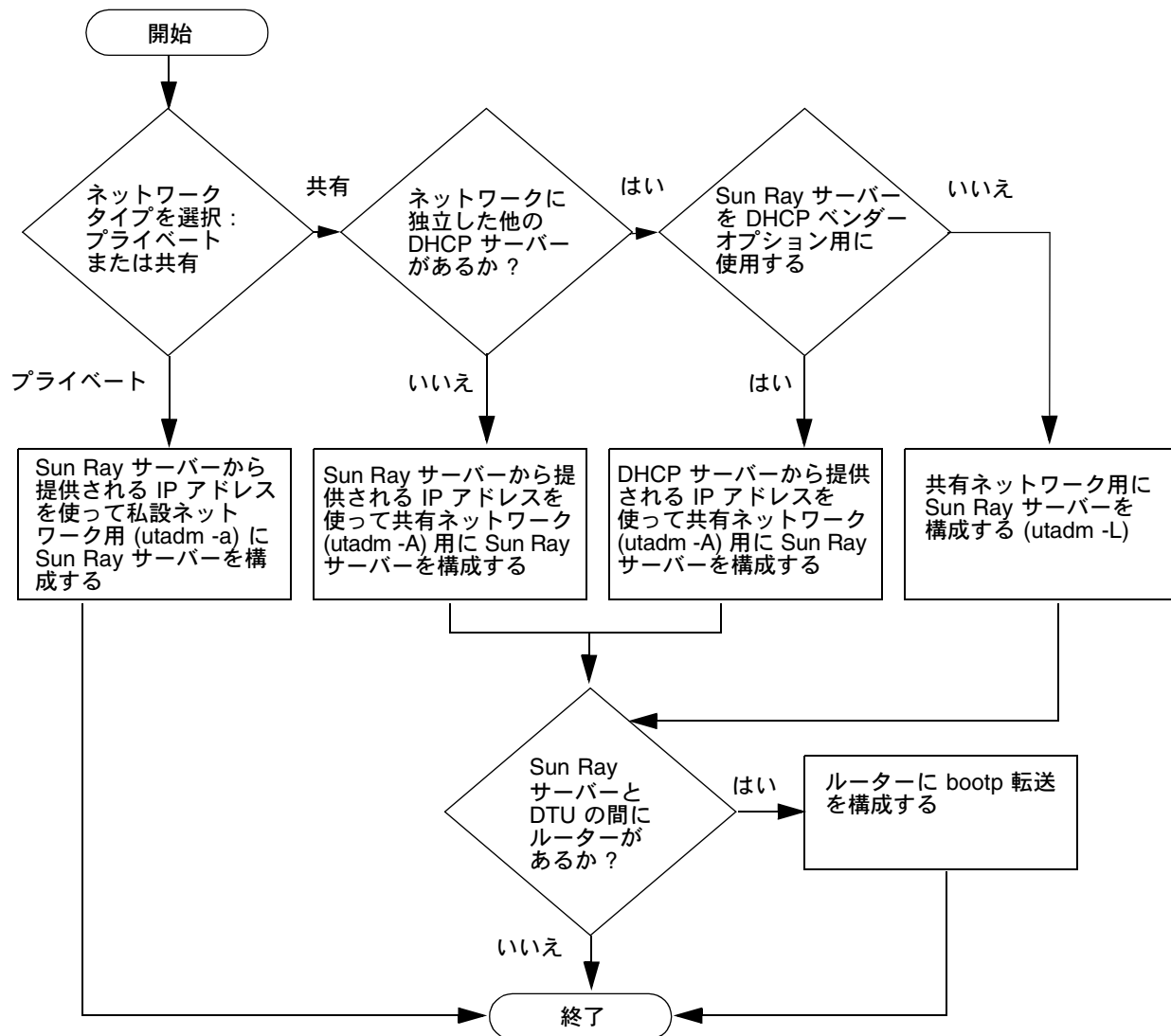
図 1-2 各種ネットワークの Sun Ray 構成
