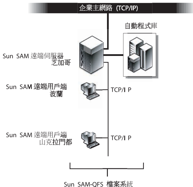
圖 7-3 Sun SAM-Remote 配置範例
