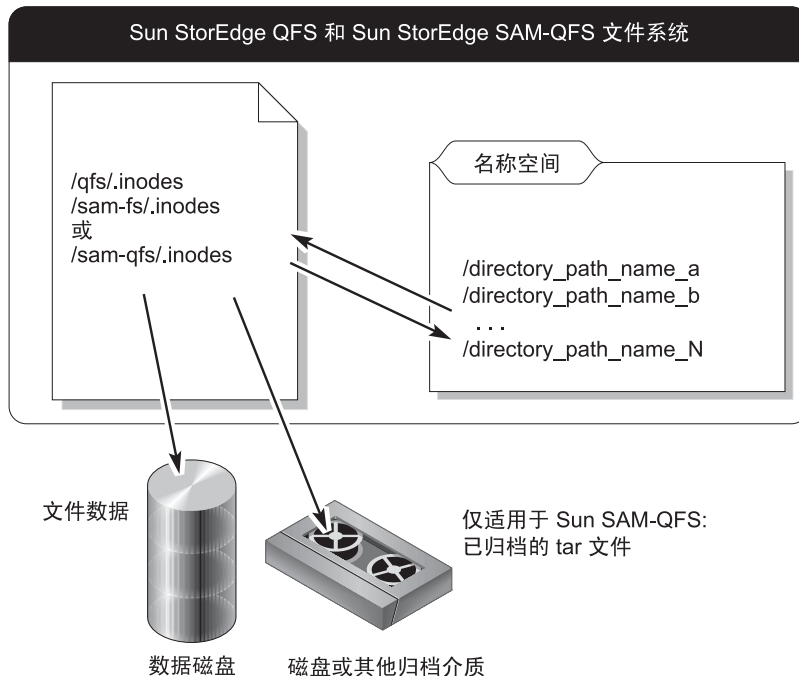
图 4-1 Sun StorageTek QFS 文件系统中的 .inodes 文件
