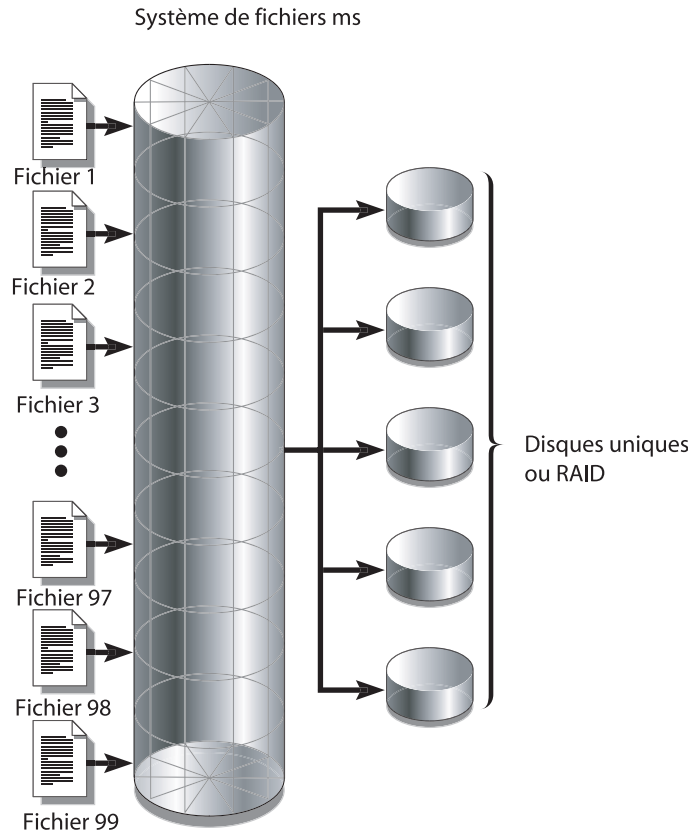
FIGURE 1-2 L'entrelacement dans un système de fichiers ms utilisant cinq périphériques
