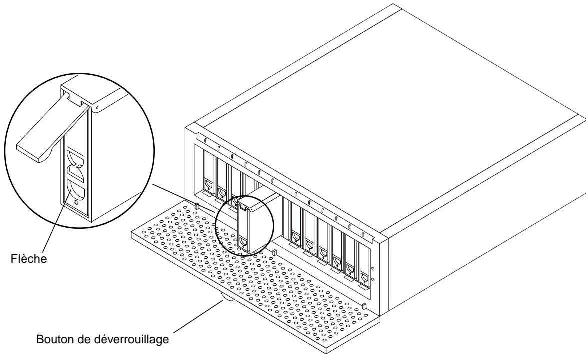
FIGURE 4-2 Retrait et remplacement d'une unité de disque
