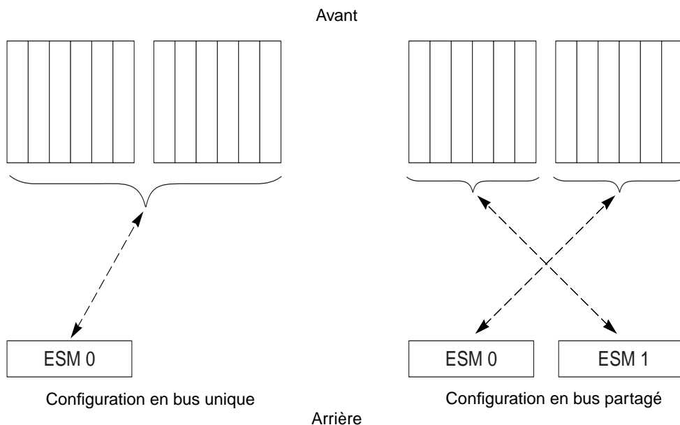
FIGURE 1-6 Disques contrôlés par un seul ESM et par deux ESM
