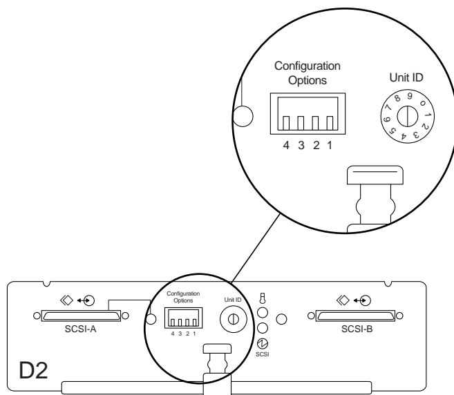
FIGURE 1-9 Bloc de commutateurs de configuration
