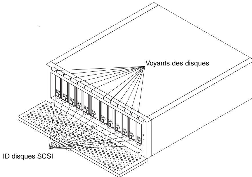
FIGURE 1-2 Vue avant de la baie de disques avec voyants des disques et ID des disques SCSI
