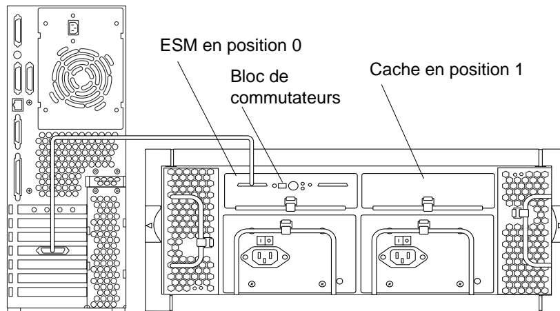
FIGURE 1-13 Configuration en bus unique avec un seul ESM, une seule carte contrôleur et un seul hôte
