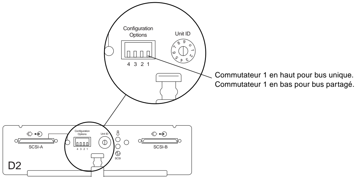
FIGURE 2-1 ESM avec commutateurs de configuration
