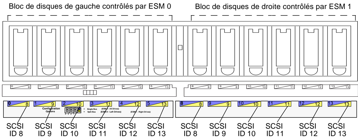
FIGURE 1-8 ID SCSI pour les disques contrôlés par deux ESM en configuration bus partagé
