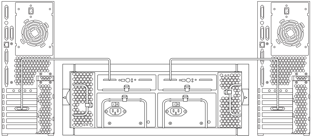
FIGURE 1-15 Configuration en bus partagé avec deux ESM et deux hôtes
