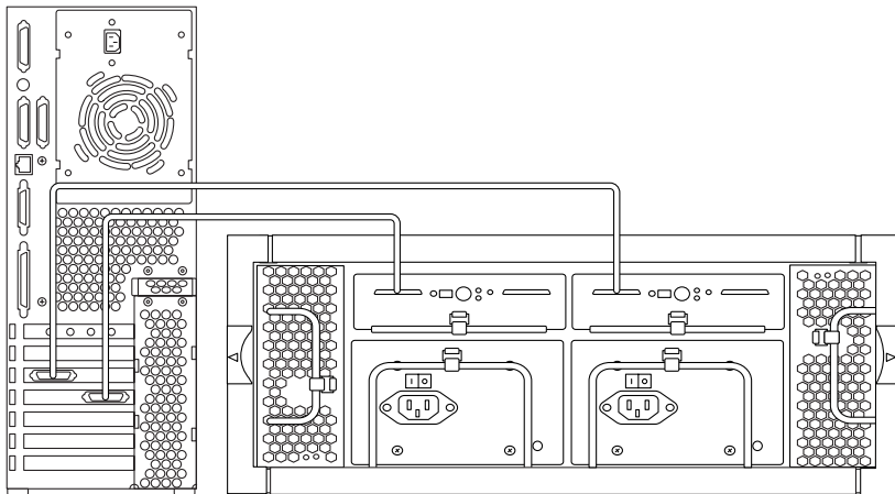
FIGURE 1-14 Configuration en bus partagé haute disponibilité avec deux ESM, deux cartes contrôleur et un seul hôte
