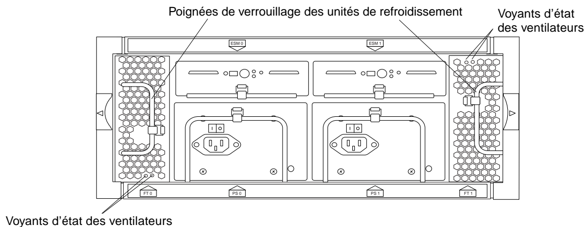
FIGURE 4-3 Unités de refroidissement
