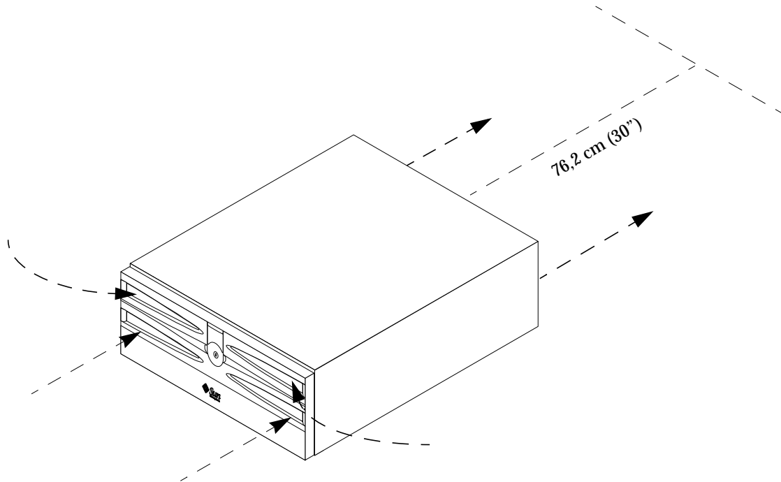
FIGURE A-1 Espace nécessaire à la circulation de l'air de la baie de disques Sun StorEdge D2
