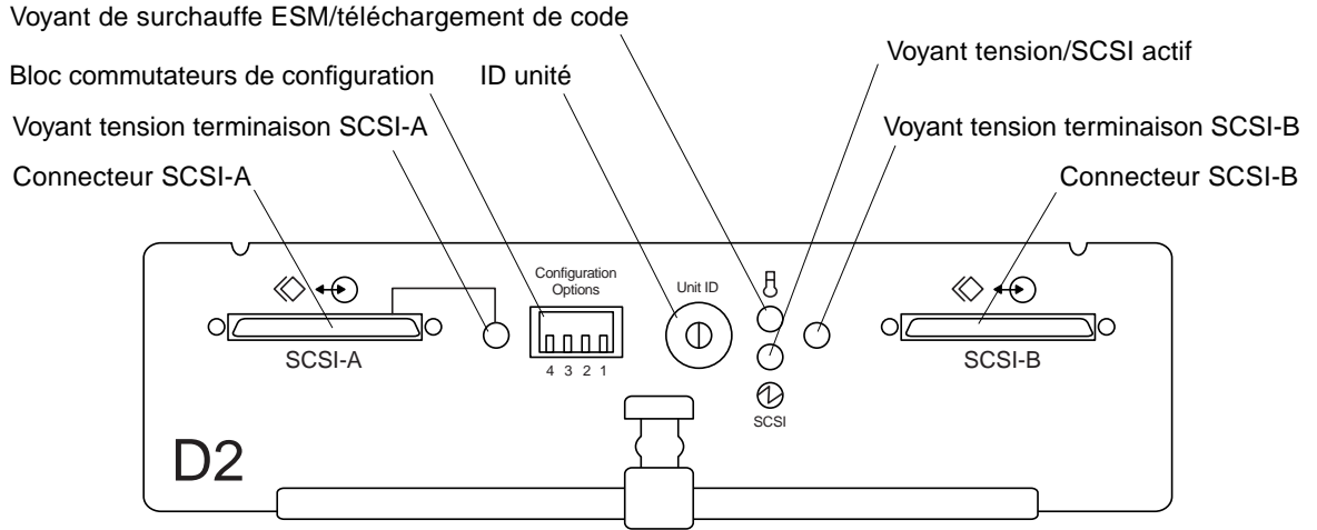
FIGURE 1-5 Avant du ESM (vu de l'arrière de la baie de disques)
