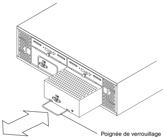
FIGURE 4-5 Retrait et remplacement d'une alimentation
