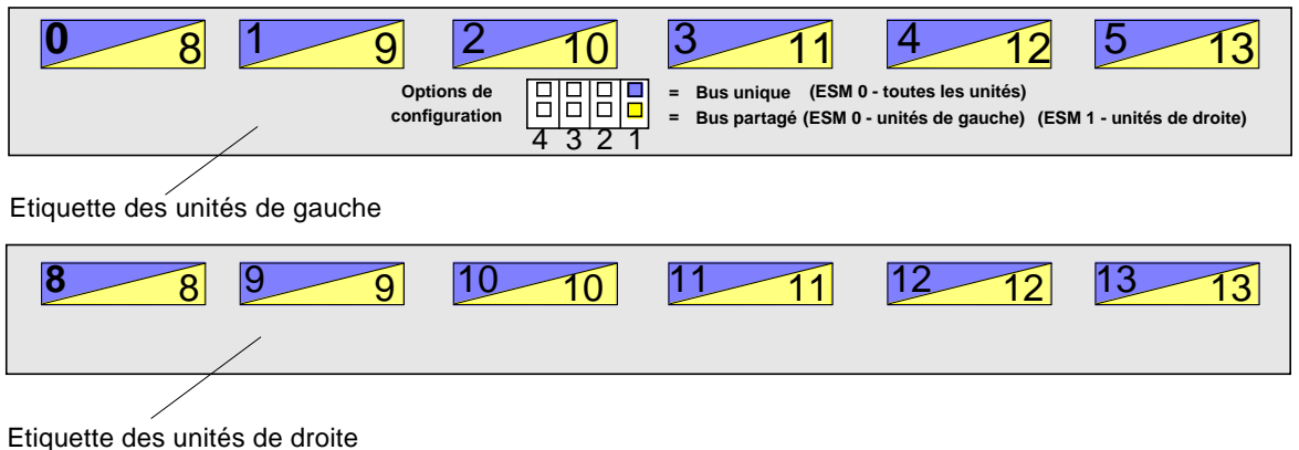
FIGURE 1-3 Etiquettes des emplacements disques avec les ID SCSI des disques
