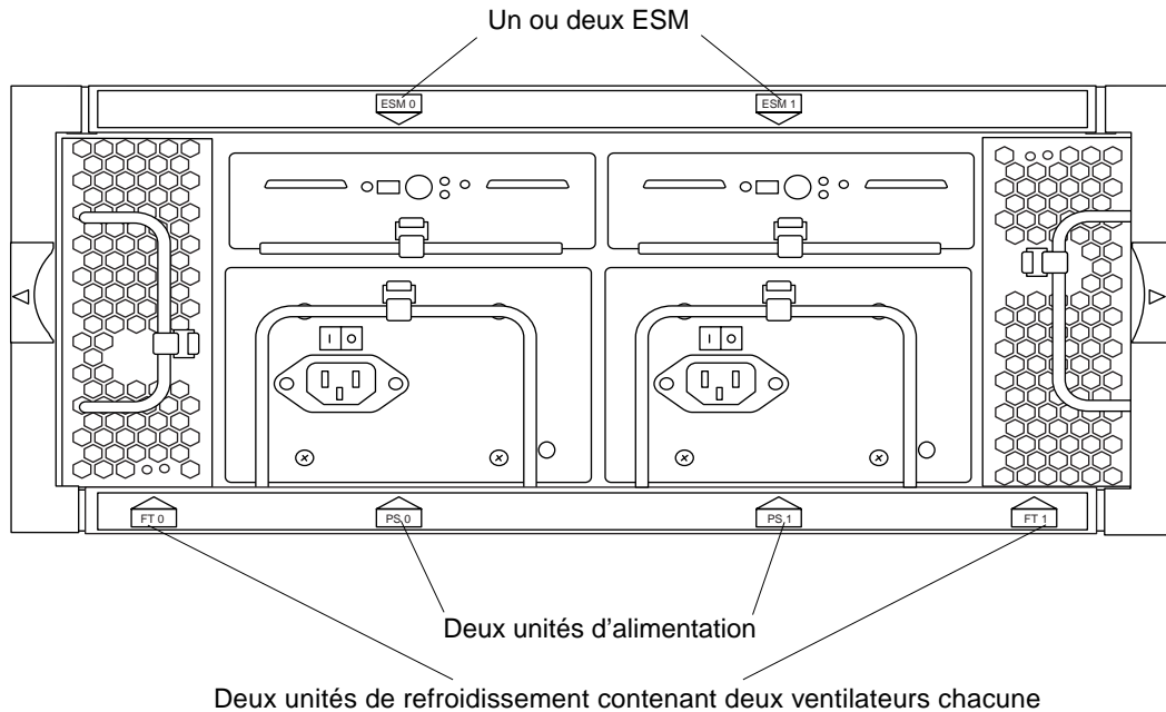
FIGURE 1-4 Vue arrière de la baie de disques avec ESM, unités d'alimentation et unités de refroidissement.
