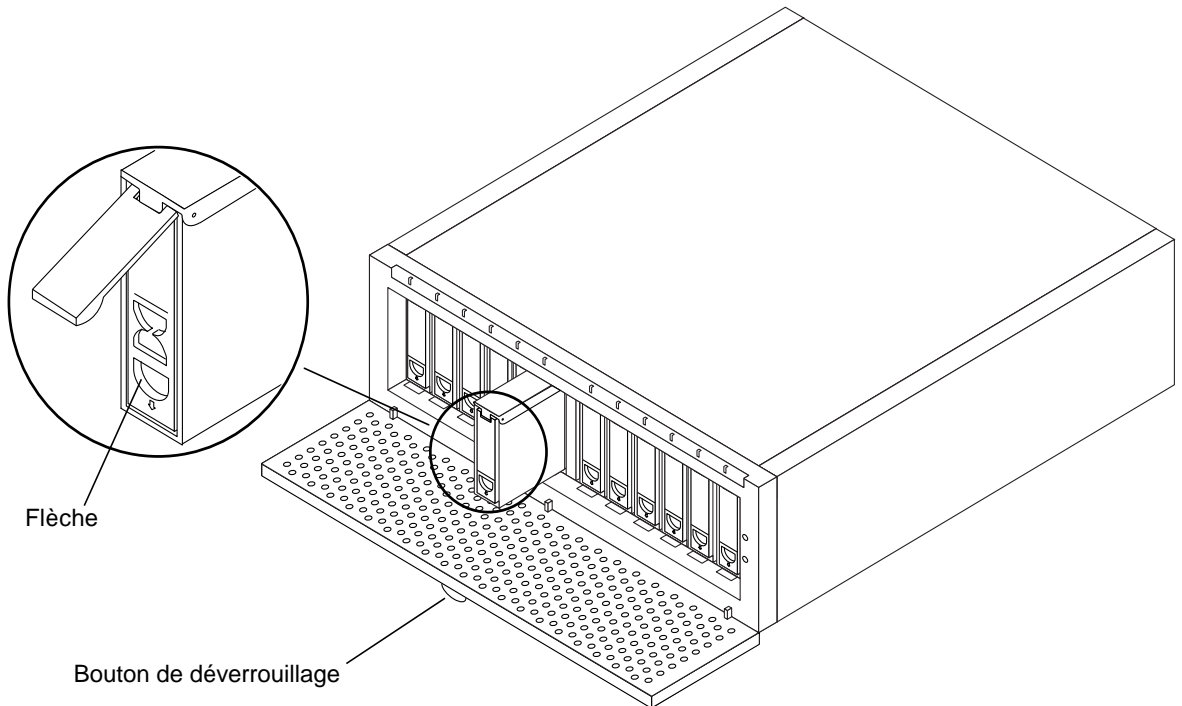
FIGURE 4-1 Retrait et remplacement d'une unité de disque
