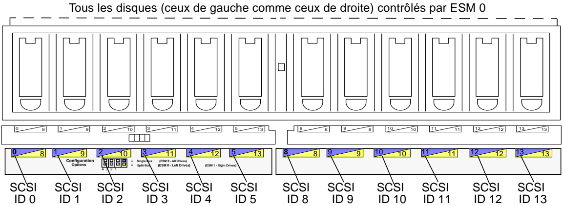
FIGURE 1-7 ID SCSI pour les disques contrôlés par un seul ESM en configuration bus unique
