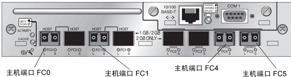
图 4-14 Sun StorEdge 3511 FC 阵列中缺省的单控制器 SFP 位置
