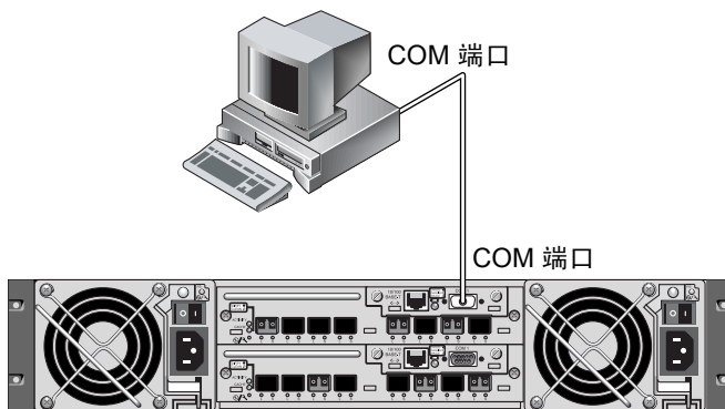
图 I-1 RAID 阵列 COM 端口在本地连接到主机系统的串行端口
