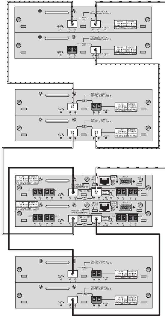
图 19 带有三个扩展单元的 Sun StorEdge 3510 FC 阵列配置
