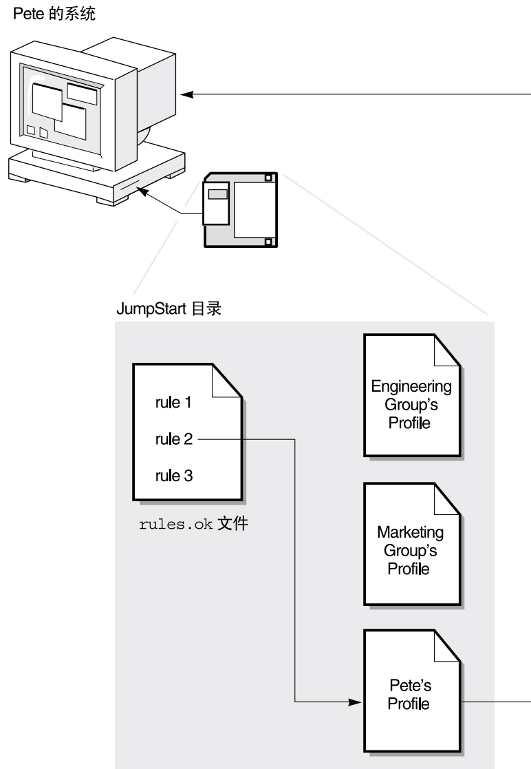
图 5-1 自定义 JumpStart 安装的工作原理：非联网示例
