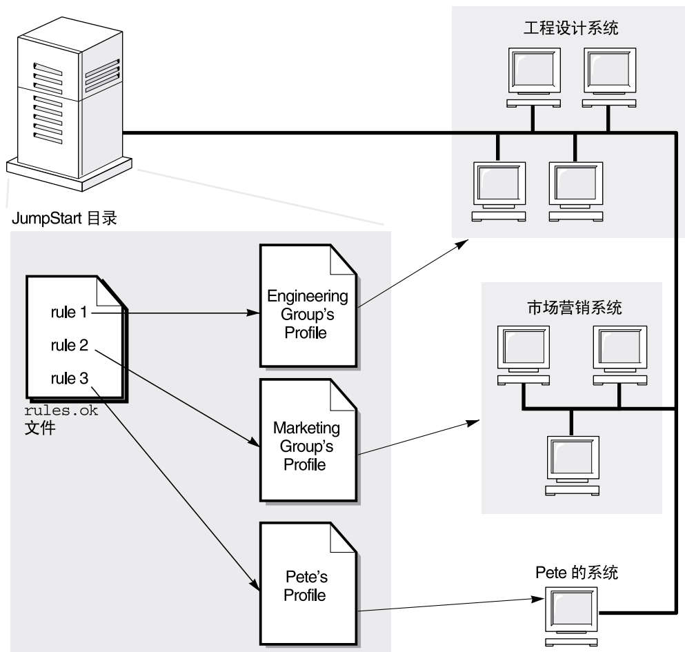
图 5-2 自定义 JumpStart 安装的工作原理：联网示例
