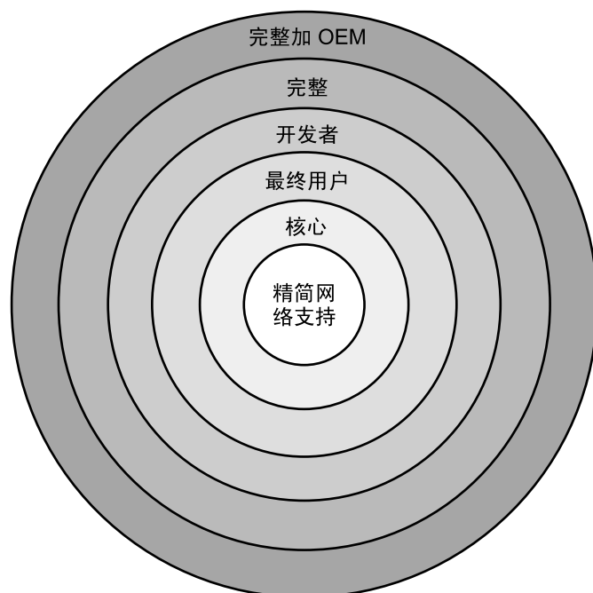
图 3-1 Solaris 软件组
