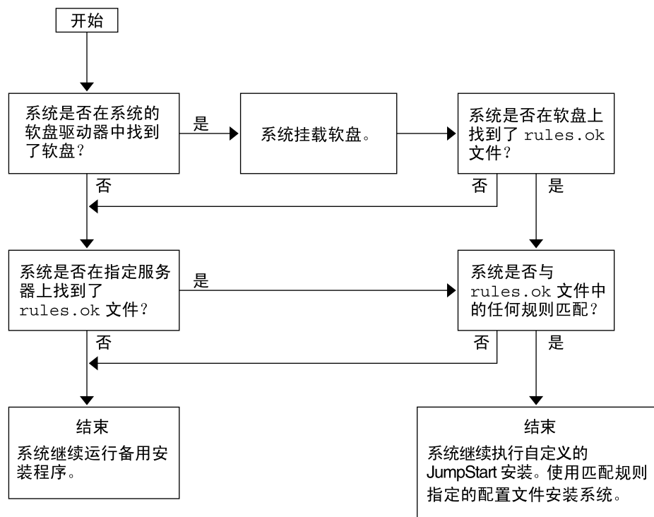
图 5-3 自定义 JumpStart 安装过程中执行的操作
