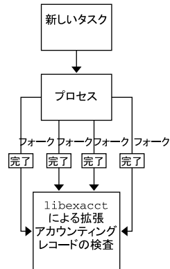
図 4-1 拡張アカウントティング起動時のタスクの追跡
