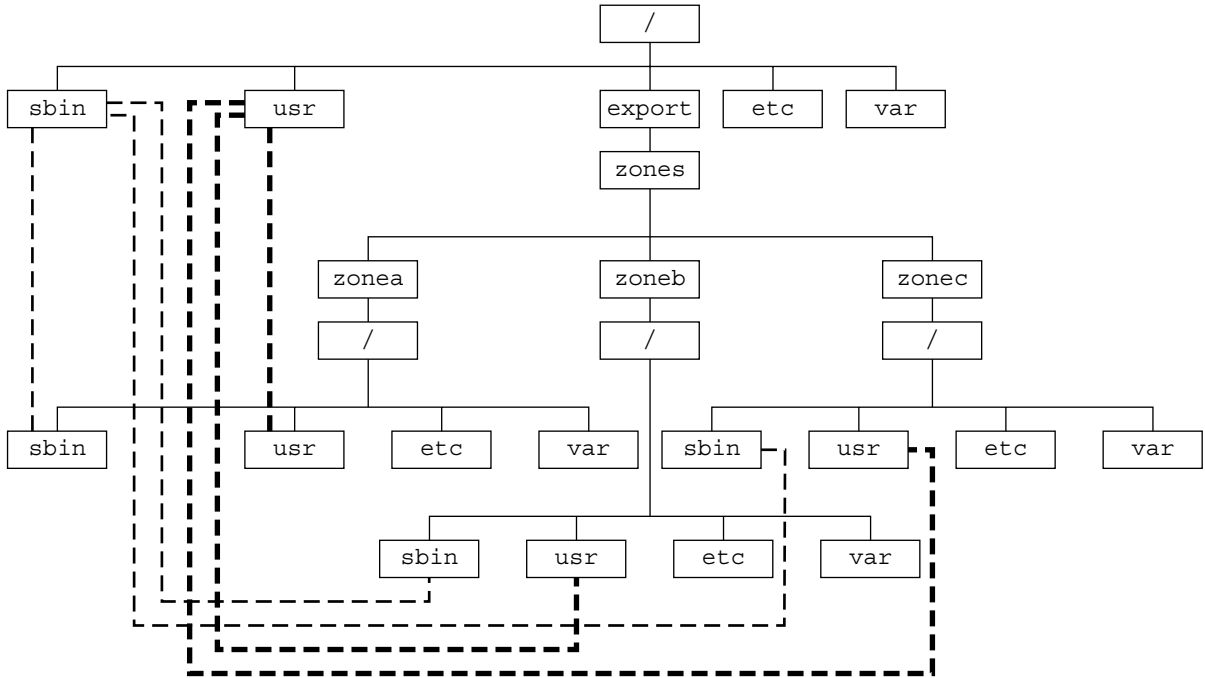
図 18-1 ループバックマウントされたファイルシステム
