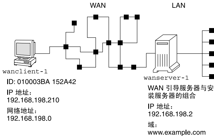
图 15-1 WAN Boot 安装的样例站点
