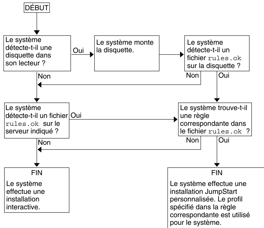
FIGURE 5-3 Organigramme d'une installation JumpStart personnalisée
