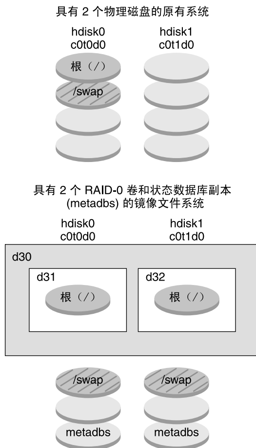
d30 – RAID-1 卷（镜像） d31 – 单片串联（子镜像） d32 – 单片串联（子镜像） 图 12-2 RAID-1 卷磁盘布局
