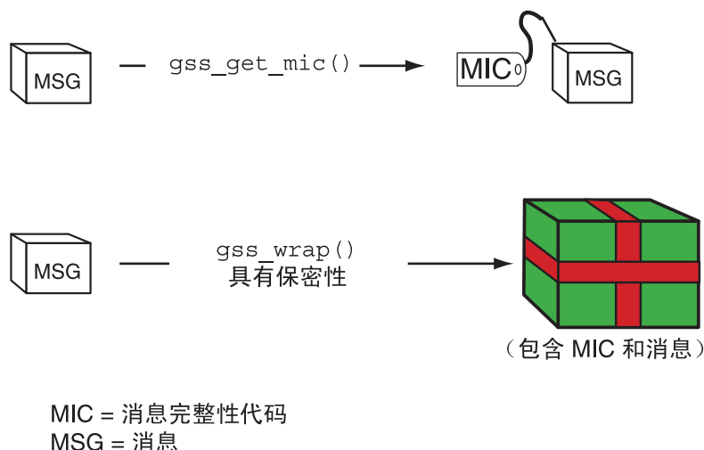
图 4-7 gss_get_mic() 与 gss_wrap()
