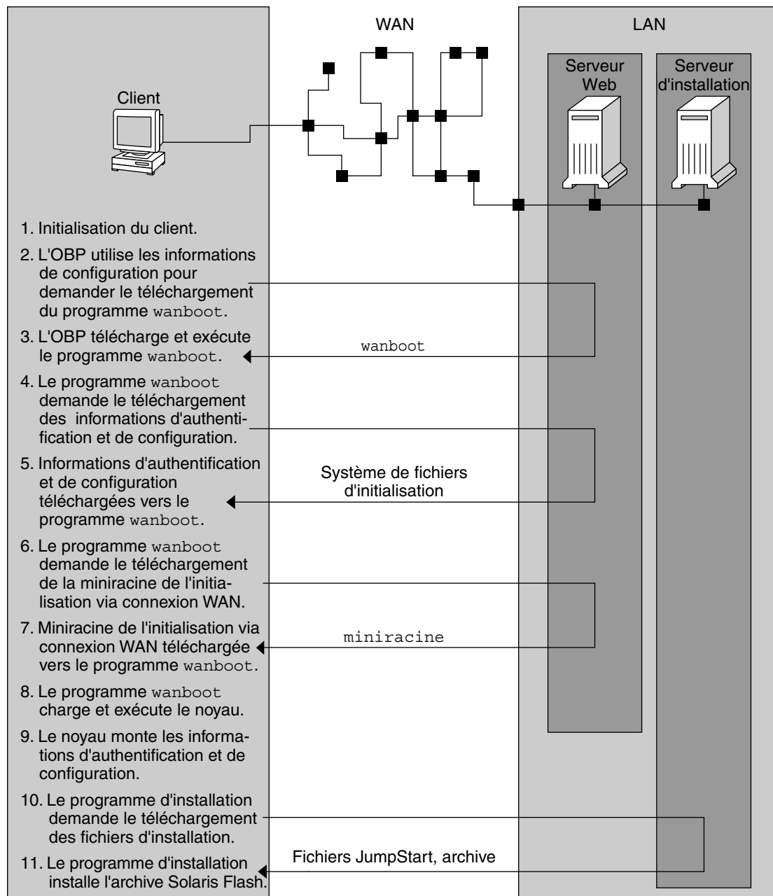
FIGURE 9-1 Déroulement des événements lors d'une installation et initialisation via connexion WAN
