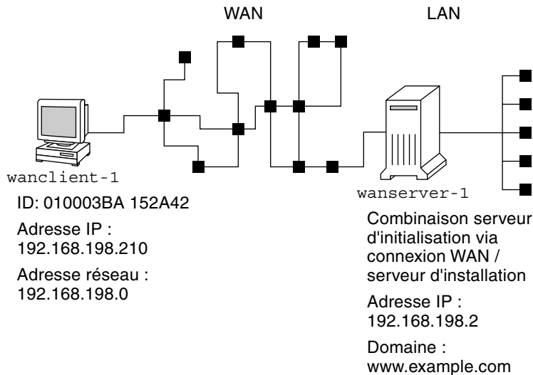
FIGURE 13-1 Exemple de configuration d'un site pour une installation et initialisation via une connexion WAN
