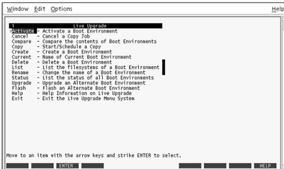
FIGURA 4-2 Menu principale di Solaris Live Upgrade
