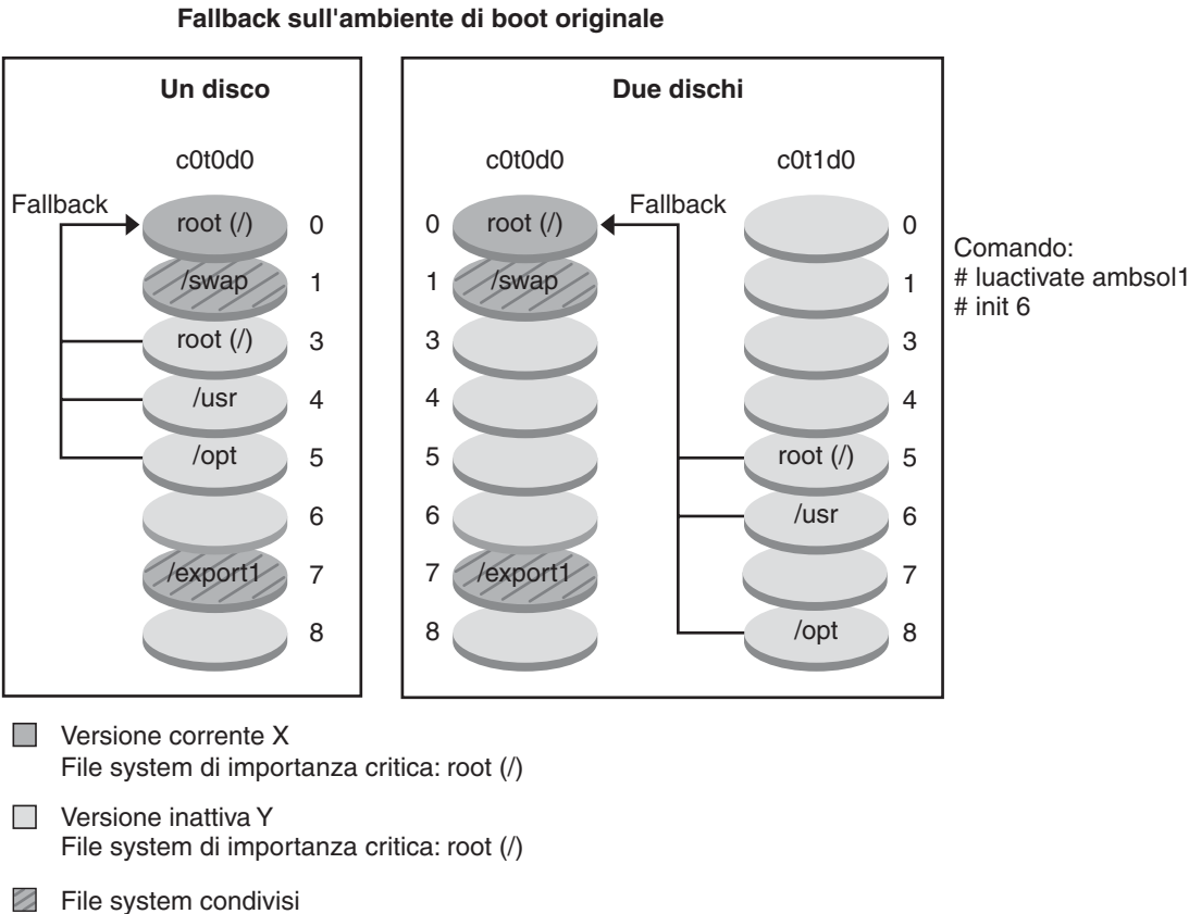
FIGURA 2-11 Ripristino dell'ambiente di boot originale
