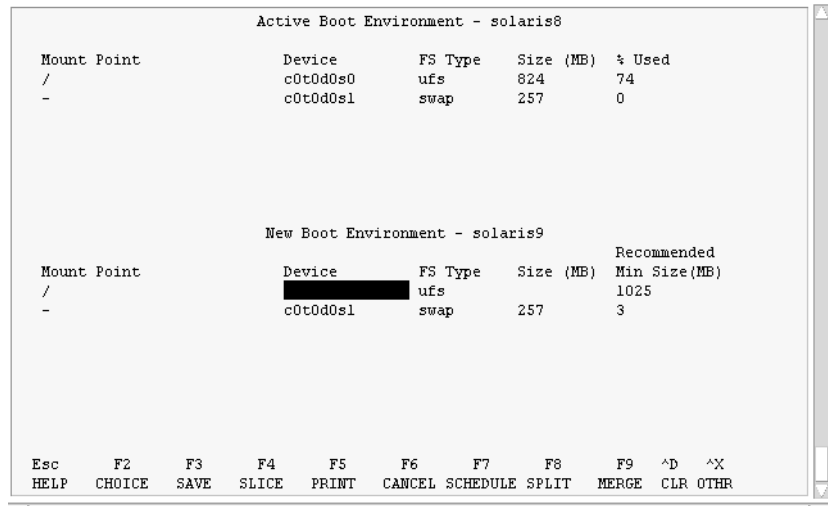
FIGURA 4-3 Menu di configurazione di Solaris Live Upgrade
