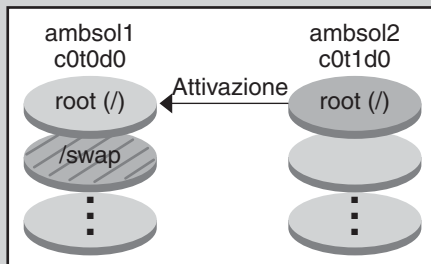
FIGURA 2-1 Processo Solaris Live Upgrade
