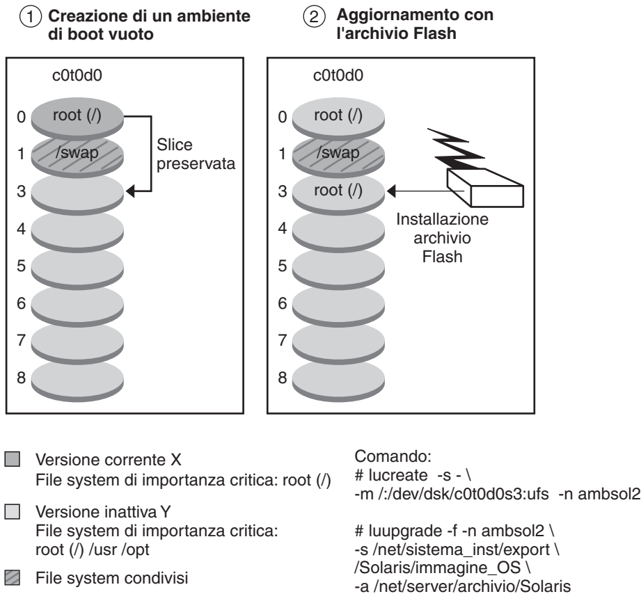
FIGURA 2–8 Installazione di un archivio Solaris Flash su un solo disco
