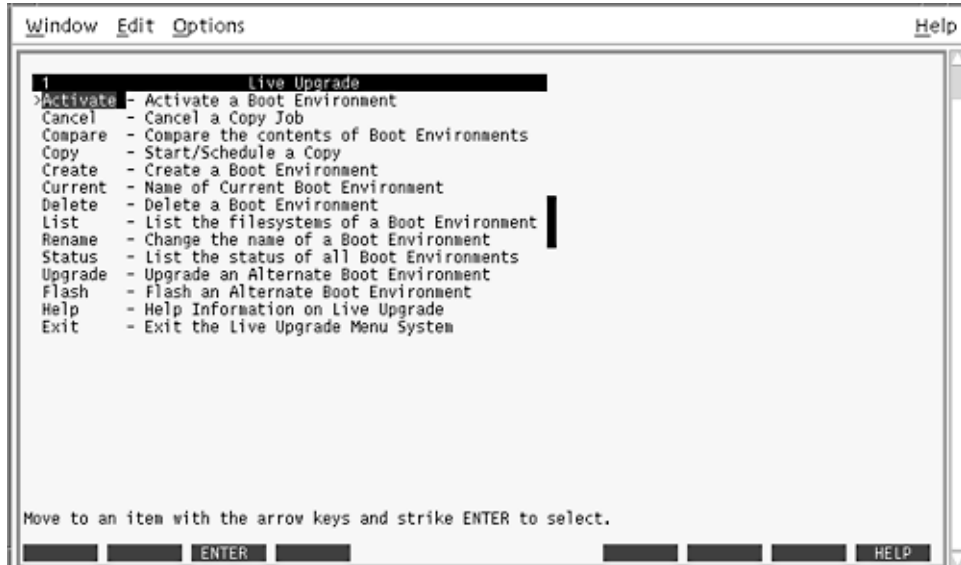
그림 4-1 Solaris Live Upgrade 기본 메뉴
