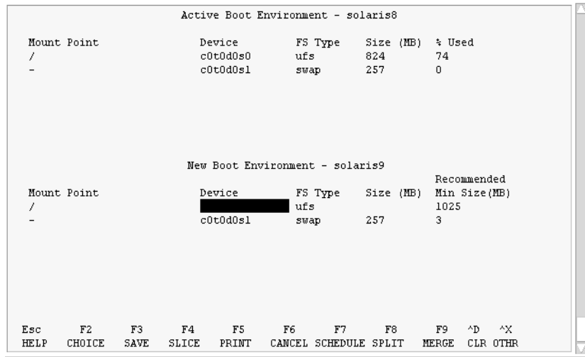
그림 4-3 Solaris Live Upgrade 구성 메뉴
