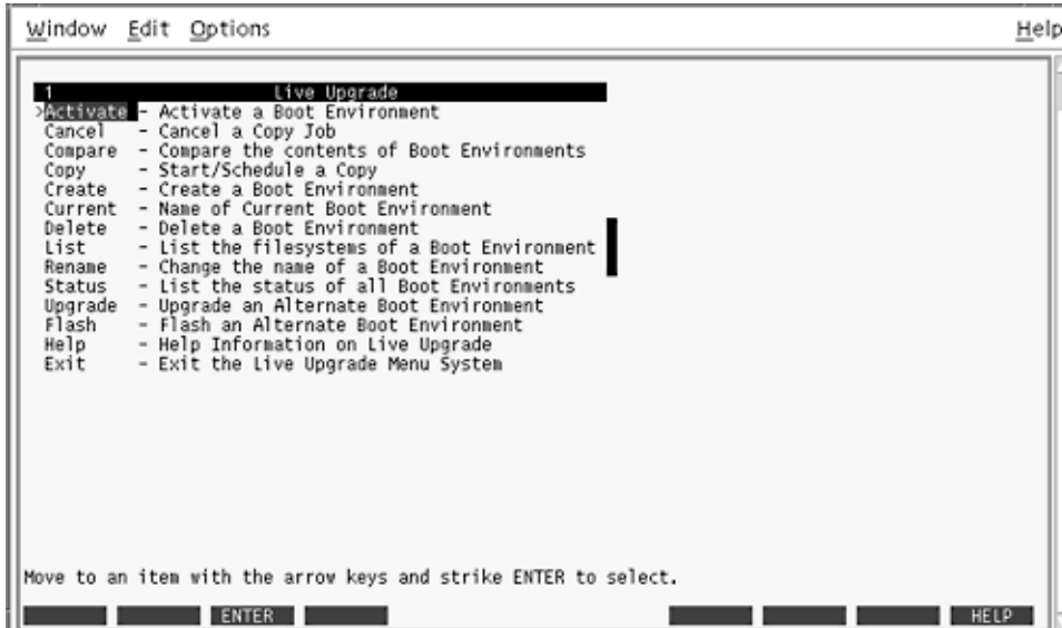
그림 4-2 Solaris Live Upgrade 기본 메뉴
