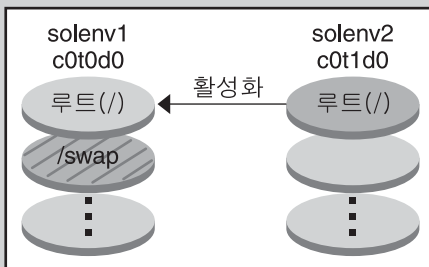
그림 2-1 Solaris Live Upgrade 프로세스
