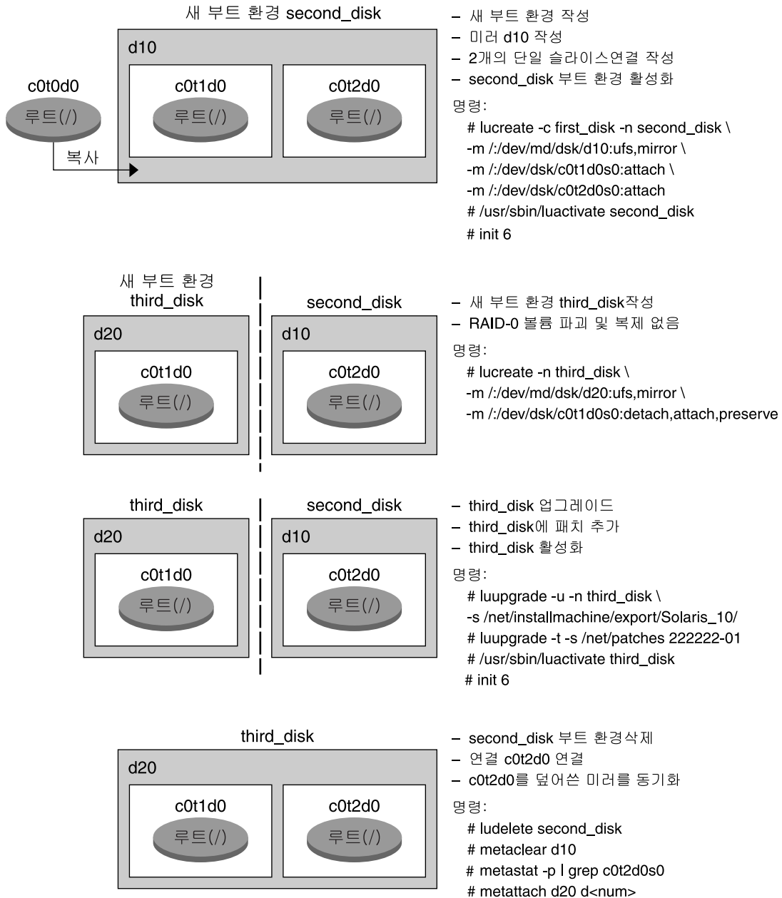
그림 9-2 RAID-1 볼륨(미러)의 한 쪽을 분리 및 업그레이드(계속)
