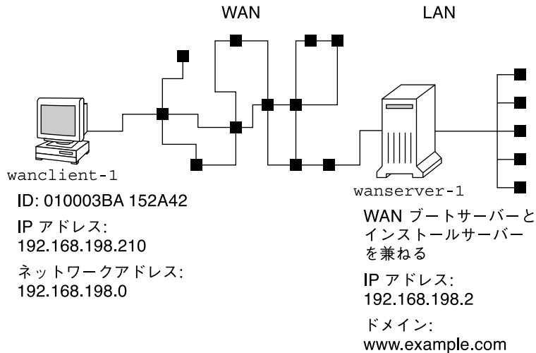
図 13-1 WANブートインストール用のサイト例
