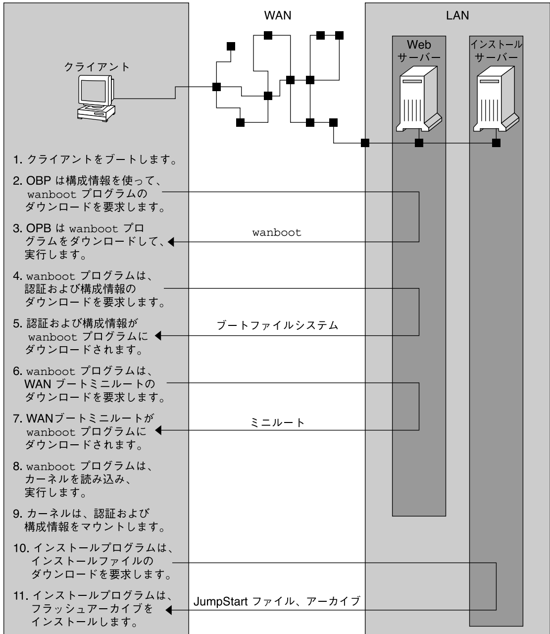
図 9-1 WANブートインストールでのイベントの順序
