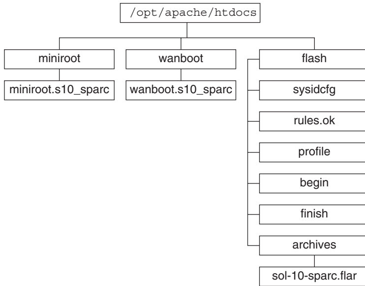
図 10-1 ドキュメントルートディレクトリの構造の例
