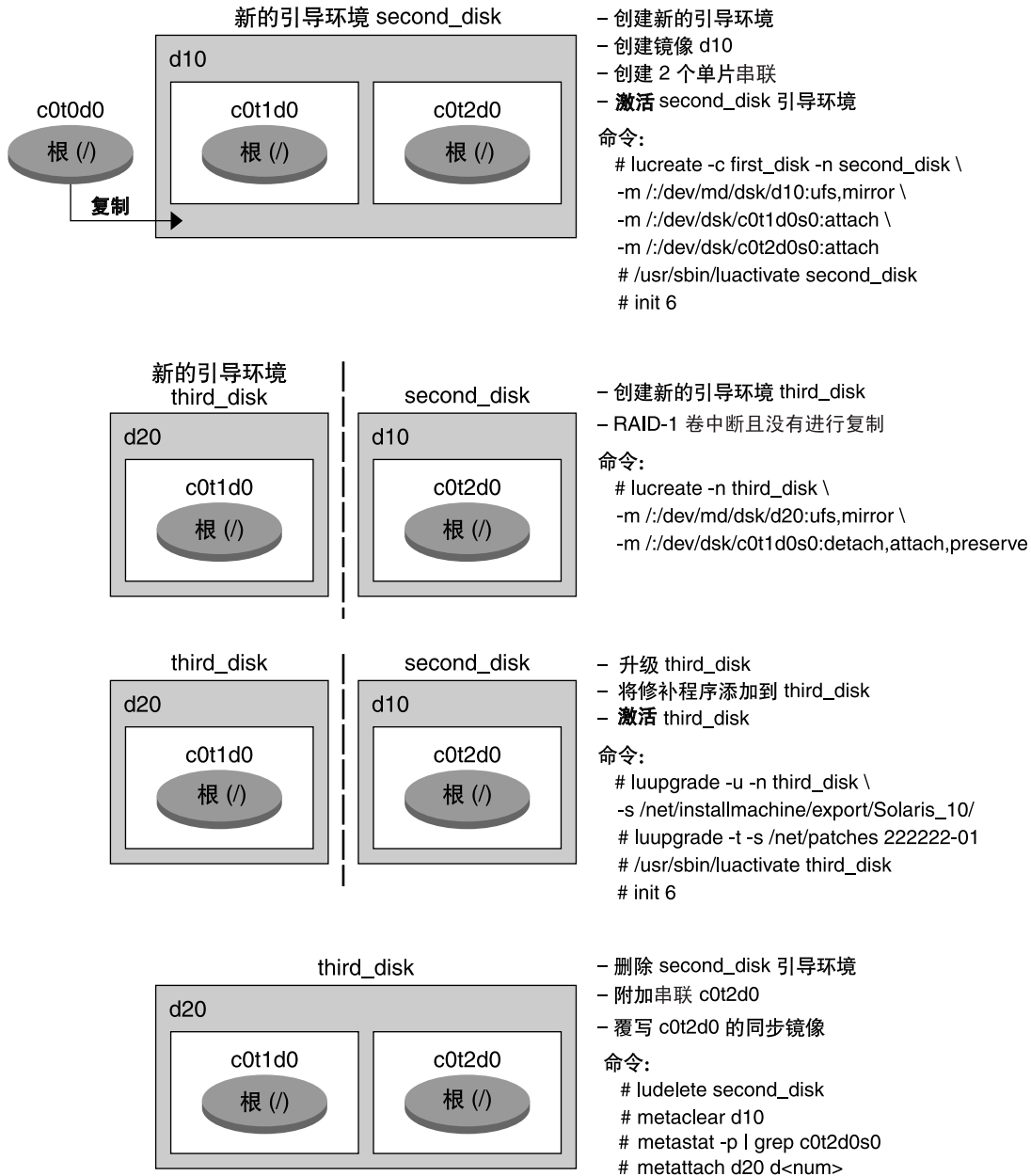
图 10-2 拆离和升级 RAID-1 卷（镜像）的一面（继续）
