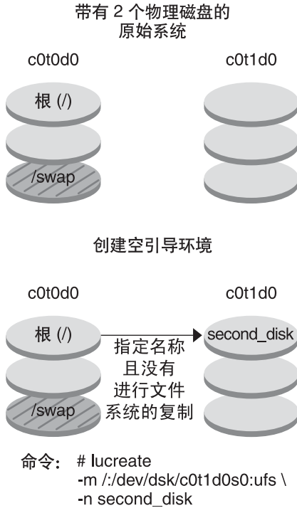
图 10-3 创建空引导环境
