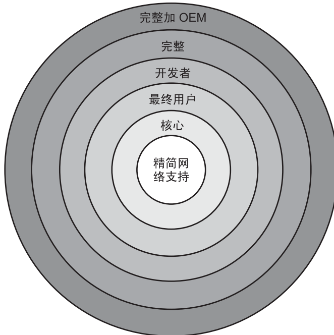
图 4-1 Solaris 软件组
