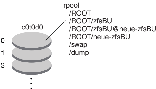
ABBILDUNG 11-2 Erstellen einer neuen Boot-Umgebung im gleichen Root-Pool
