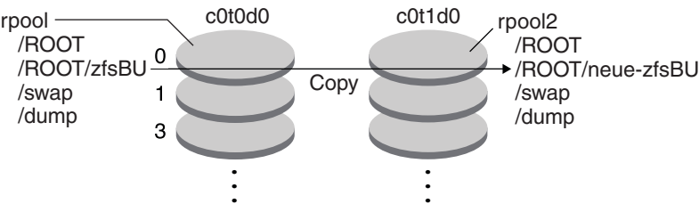
ABBILDUNG 11-3 Erstellen einer neuen Boot-Umgebung in einem anderen Root-Pool
