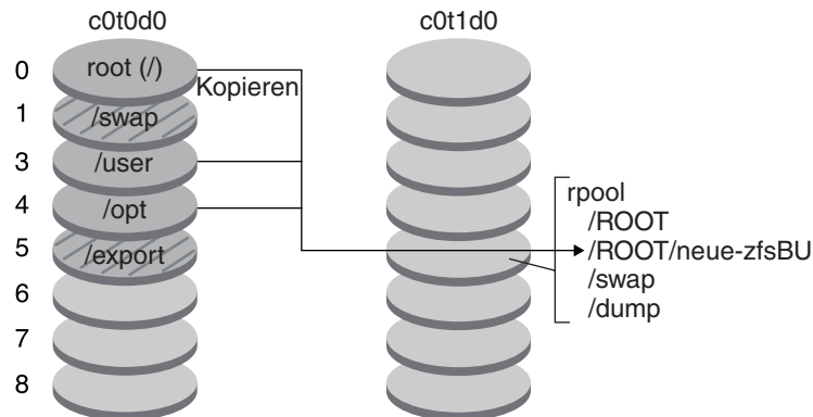
ABBILDUNG 11-1 Migration von einem UFS-Dateisystem auf ein ZFS-Root-Pool
