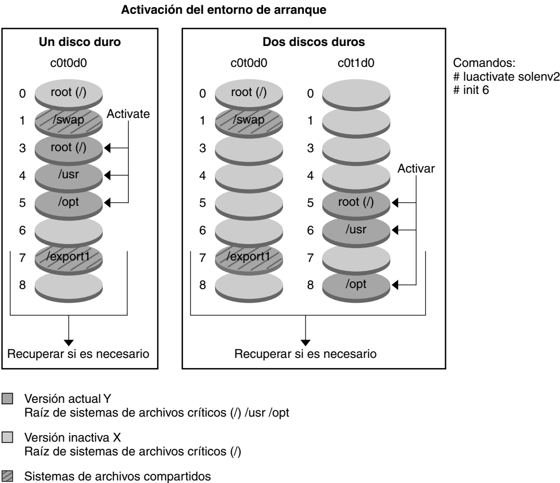
FIGURA 2–10 Activación de un entorno de arranque inactivo
