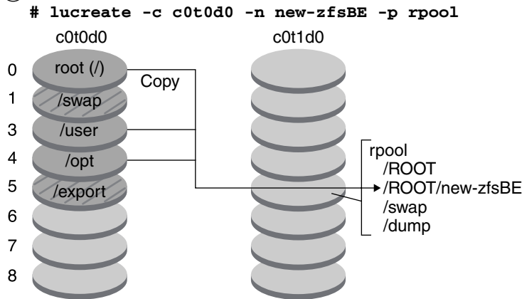
FIGURA 11-1 Migración de un sistema de archivos de UFS a una agrupación root de ZFS
