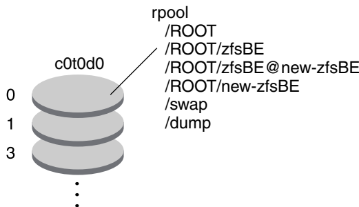
FIGURE 11-2 Création d'un environnement d'initialisation dans le même pool racine
