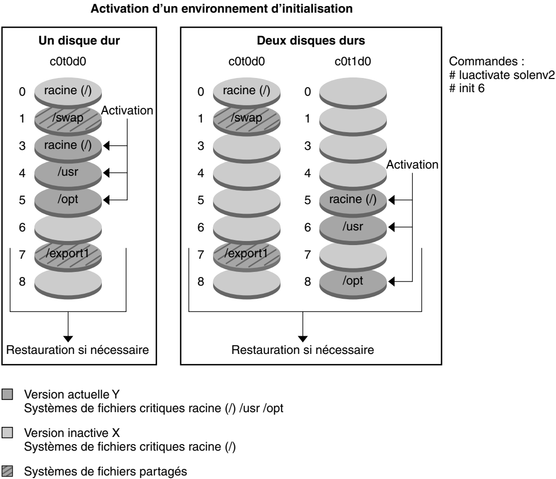
FIGURE 2–10 Activation d'un environnement d'initialisation inactif
