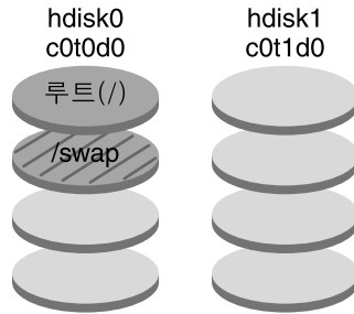
그림 9-2 RAID-1 볼륨 디스크 레이아웃
