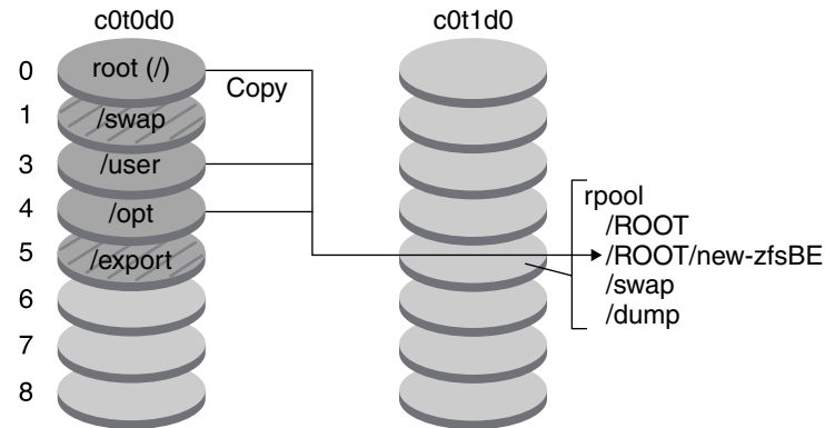
EXEMPLE 11-1 Migration d'un système de fichiers racine (/) UFS vers un pool racine ZFS
