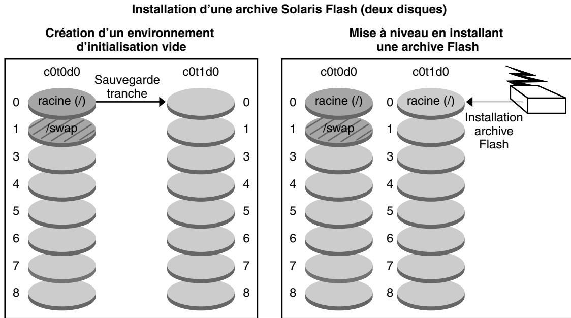
FIGURE 2-9 Installation d'une archive Solaris Flash sur deux disques
