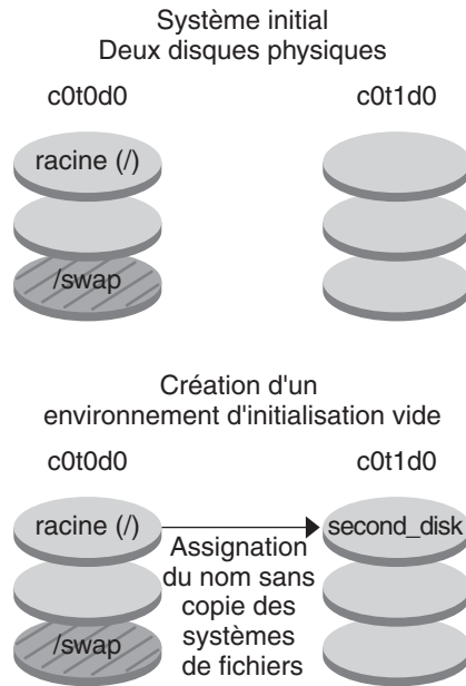
FIGURE 9-3 Création d'un environnement d'initialisation vide
