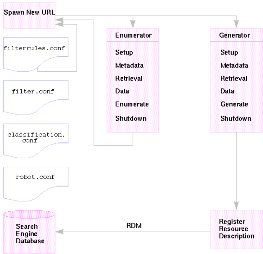
图 11-1 Robot 的工作机理
