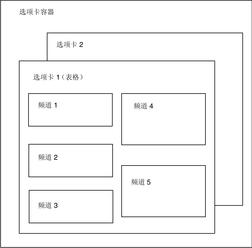
图 5-1 门户桌面容器层次结构示例
