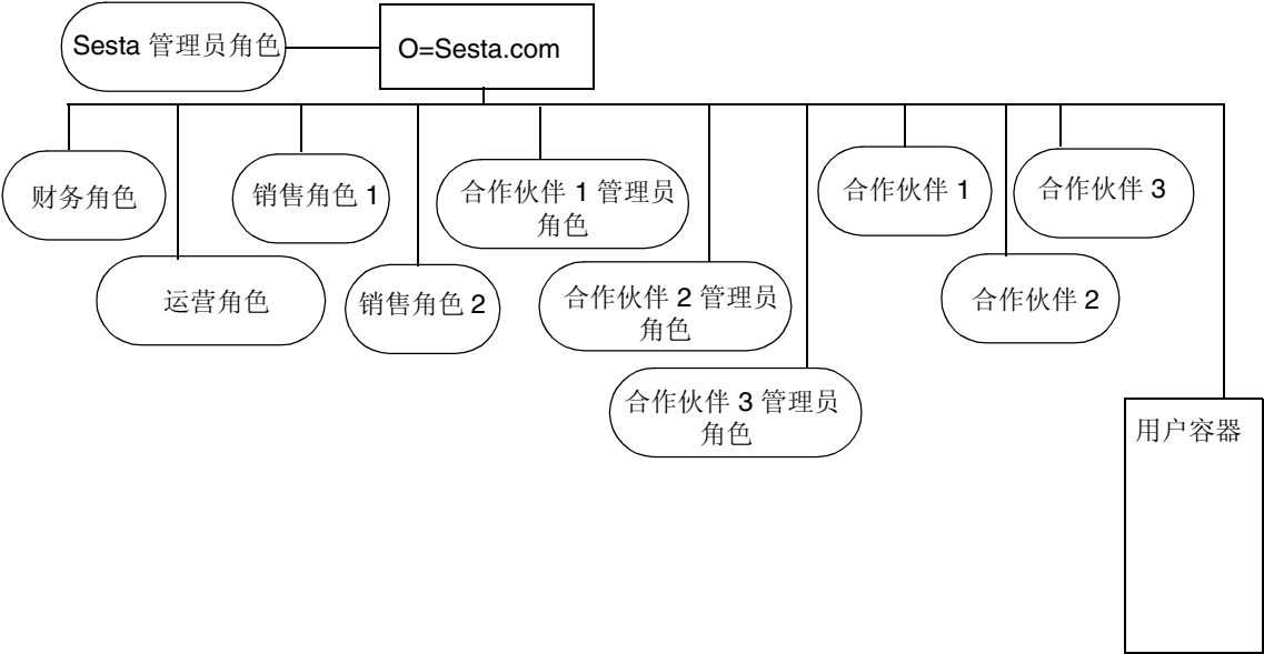
图 3-2 平列式目录结构
