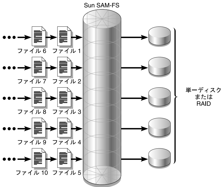
図 2-1 5 つの装置を使用するラウンドロビン式の Sun SAM-FS ファイルシステム
