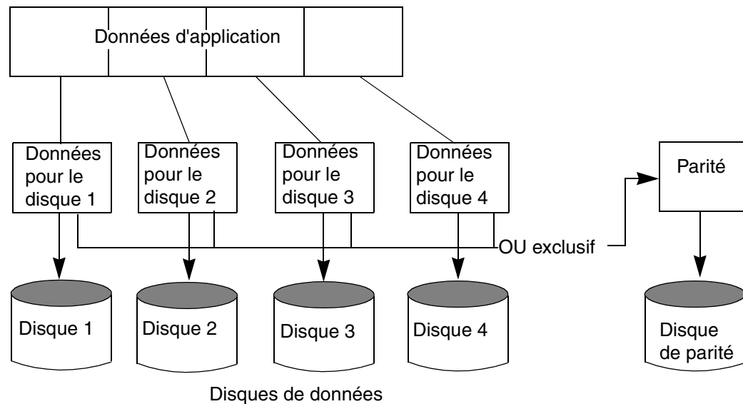
Figure 3. Écriture de données sur RAID 3
