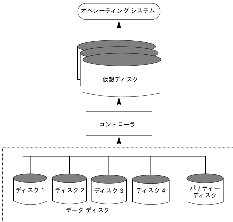
図2. RAID-3 ディスクアレイ
