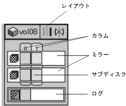
図4. [オブジェクト表示]ウィンドウ内のボリューム
