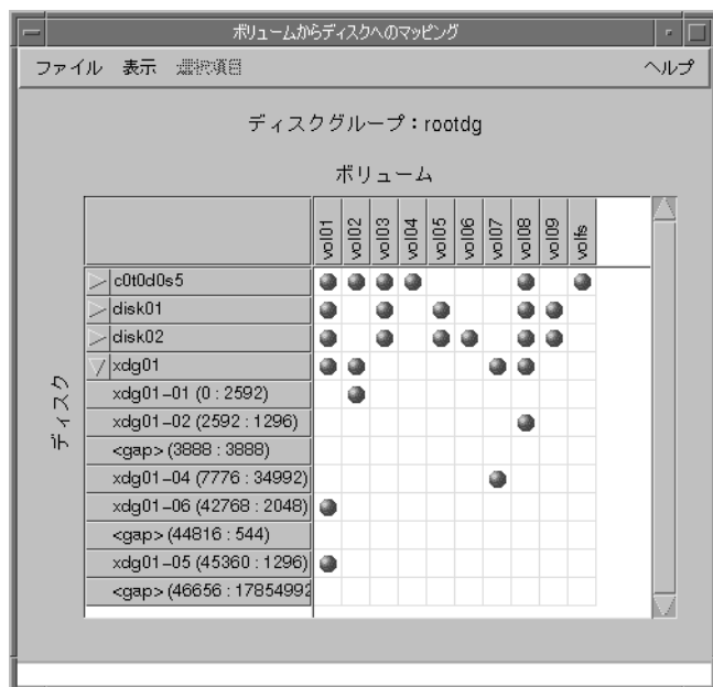
図 6. [ ボリュームからディスクへのマッピング ] ウィンドウ
