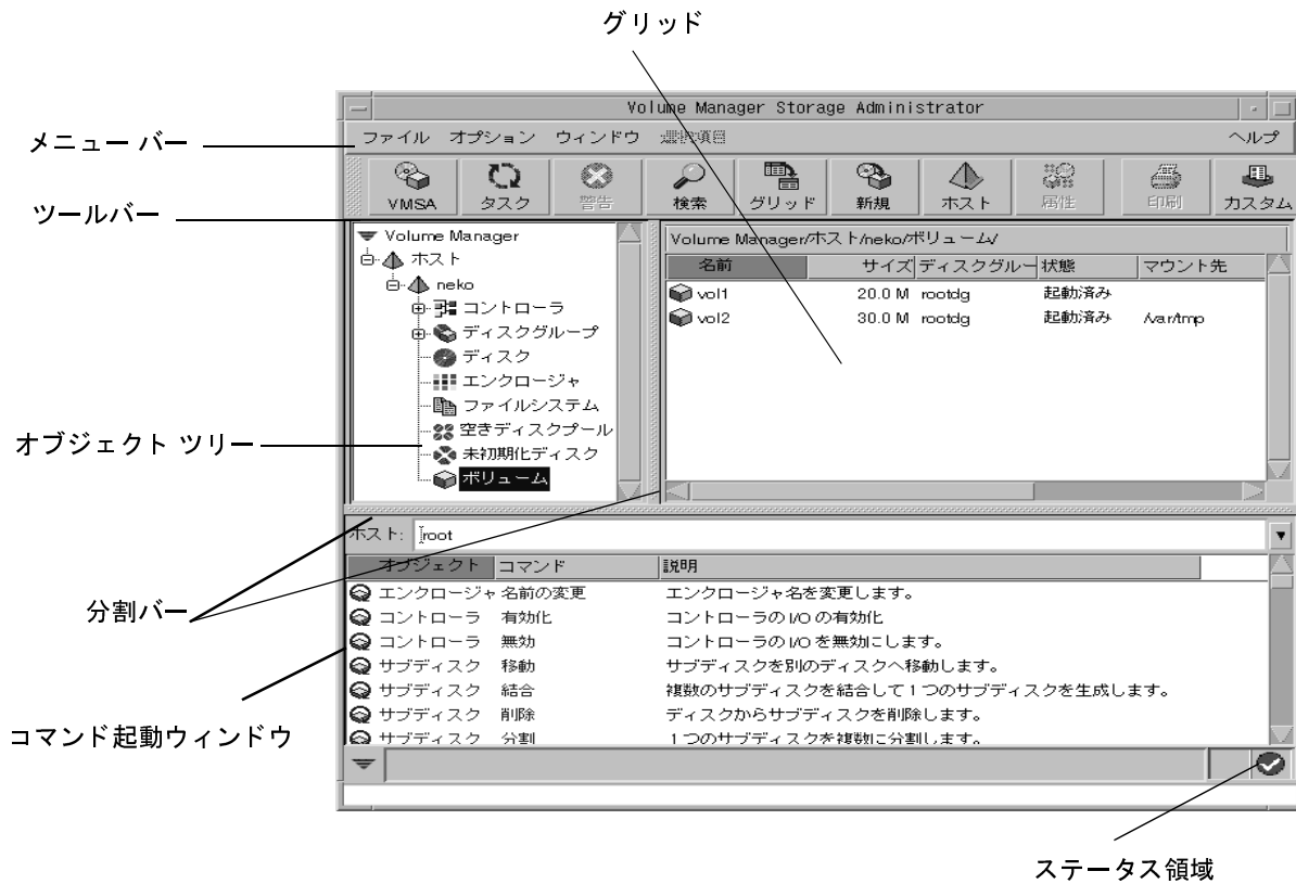
図 1. メイン ウィンドウ
