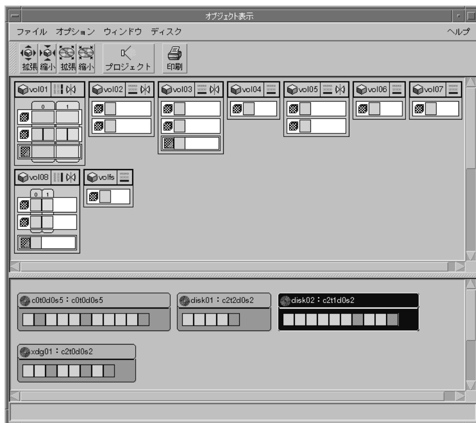
図 3. [ オブジェクト表示 ] ウィンドウ
