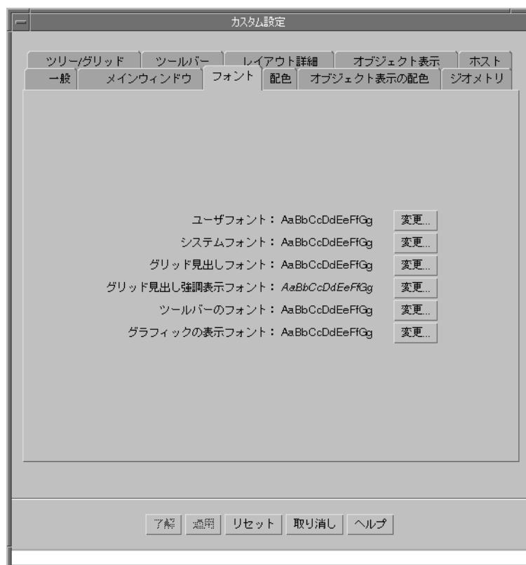
図 14. [カスタム設定]ウィンドウ
