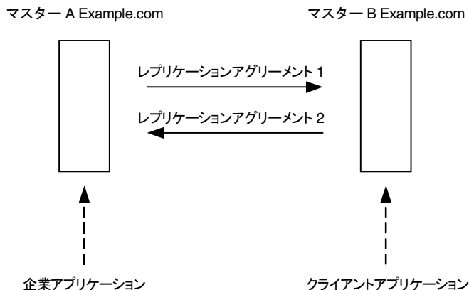
図 6-9 ロードバランスのためのマルチマスターレプリケーションの使用
