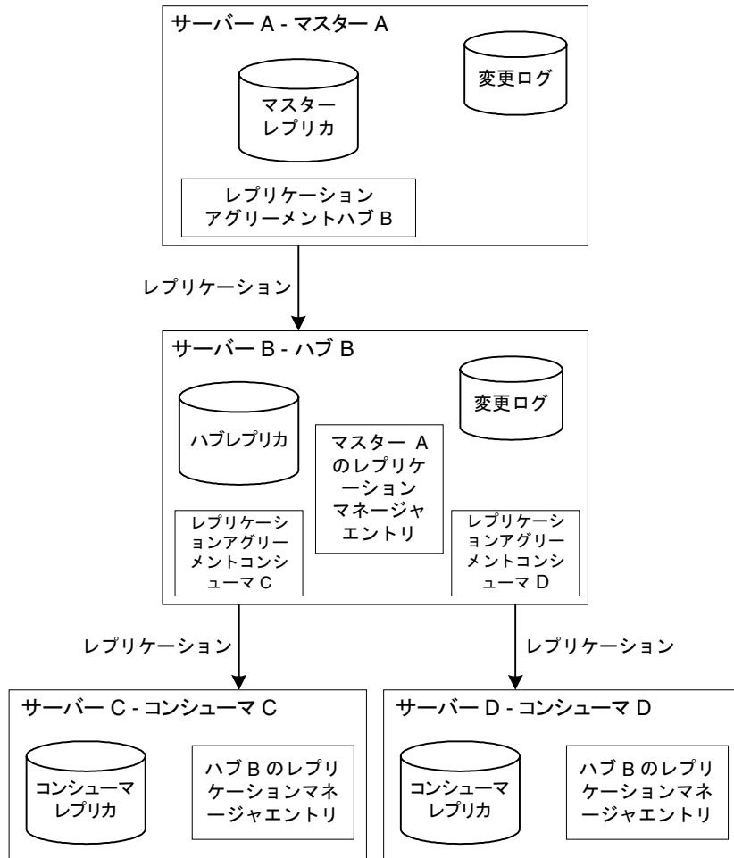
図 6-7 カスケード型レプリケーションのサーバー設定
