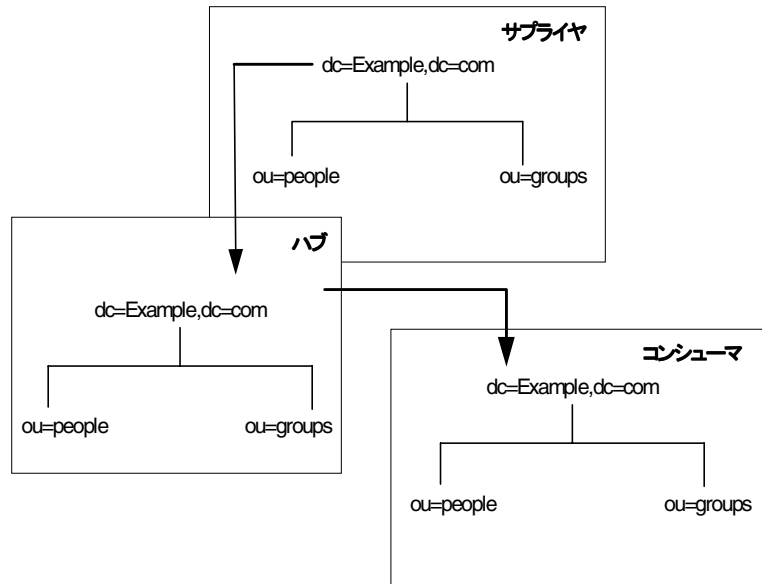
図 6-6 カスケード型レプリケーション設定
