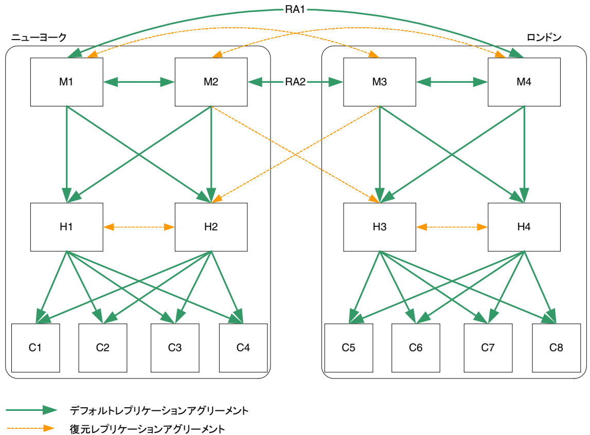
図 9-10 2つのデータセンターの復元レプリケーションアグリーメント
