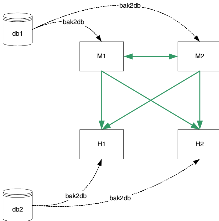
図 9-3 バイナリ復元
