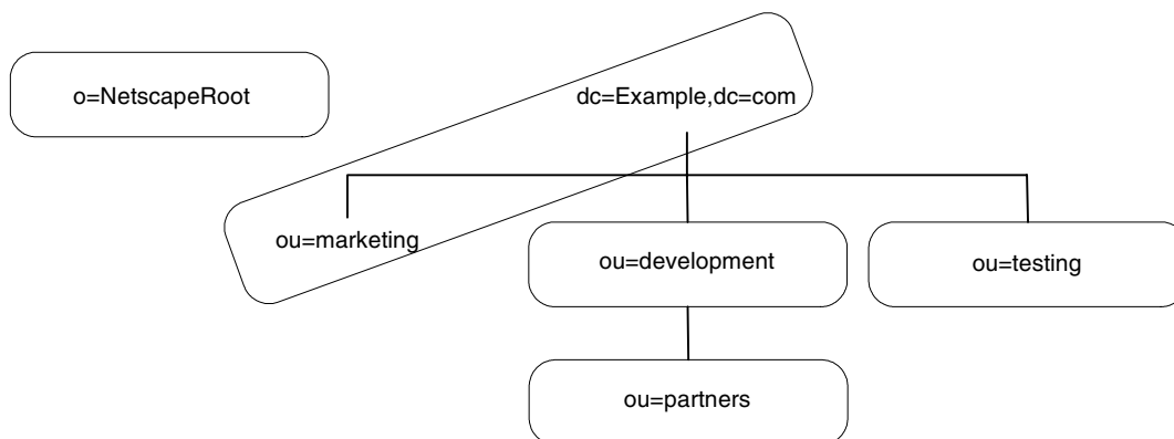
図 5-5 5 つのデータベースに分割された Example.com 社のディレクトリツリー
