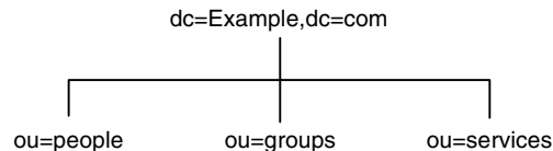
図 5-1 3つのサブサフィックスを持つディレクトリツリー
