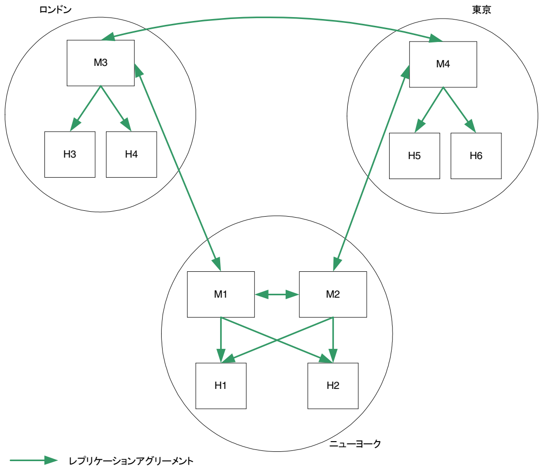
図 9-11 3つのデータセンターの基本トポロジ
