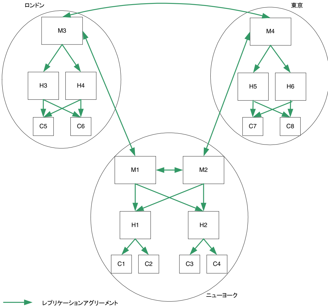
図 9-12 読み取りパフォーマンスのための3つのデータセンターのスケーリング
