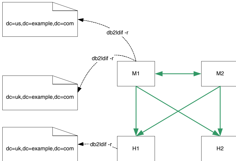
図 9-2 db2ldif -r によるバックアップ
