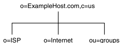
図 4-5 ISP ExampleHost.com のディレクトリ情報ツリー
