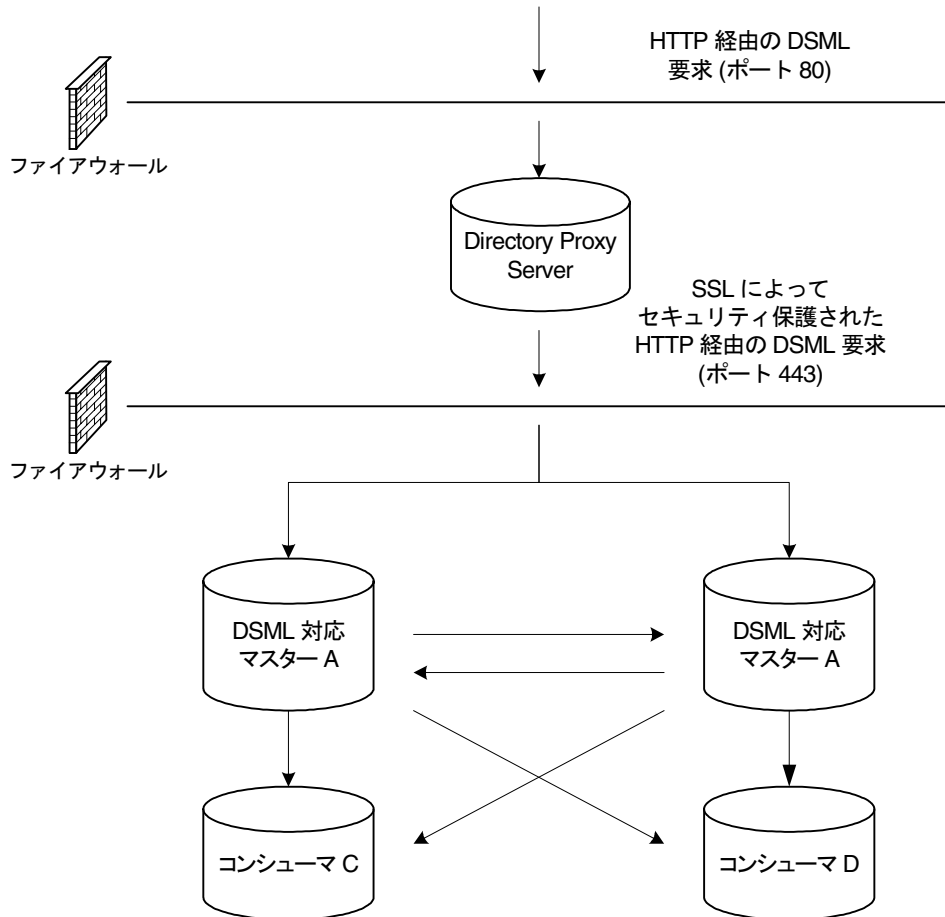
図 2-1 DSML 対応のディレクトリの配備例
