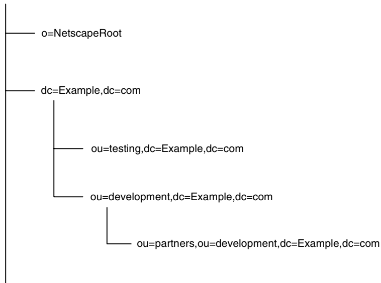
図 5-6 Example.com 社のサフィックスと関連エン트리
