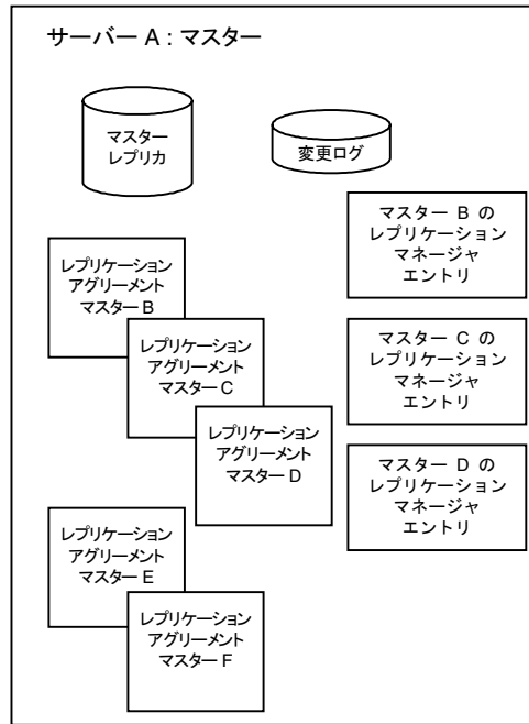
図 6-4 マスター A のレプリケーション設定 (完全にメッシュ化されたトポロジ)
