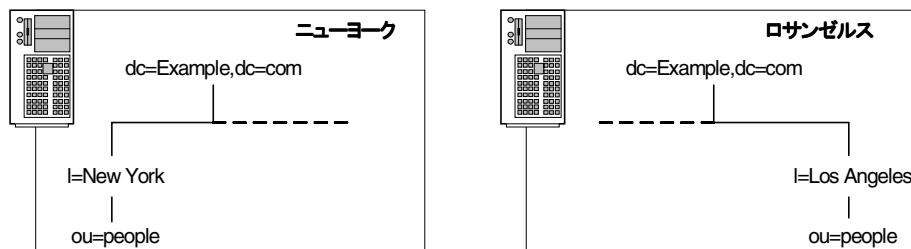
図 6-10 ニューヨークとロサンゼルスでそれぞれにあるサブツリー
