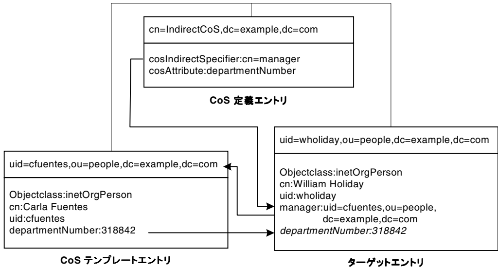
図 4-13 間接 CoS の定義とテンプレートの例
