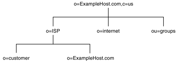
図 4-10 ExampleHost.com のディレクトリ情報ツリー
