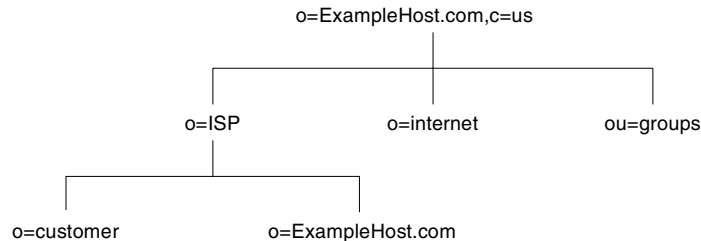
図 4-7 ExampleHost.com 社のインターネットホストディレクトリ情報ツリー
