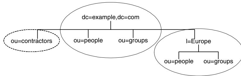
図 4-2 複数のサブサフィックスを持つ単一のルートサフィックス
