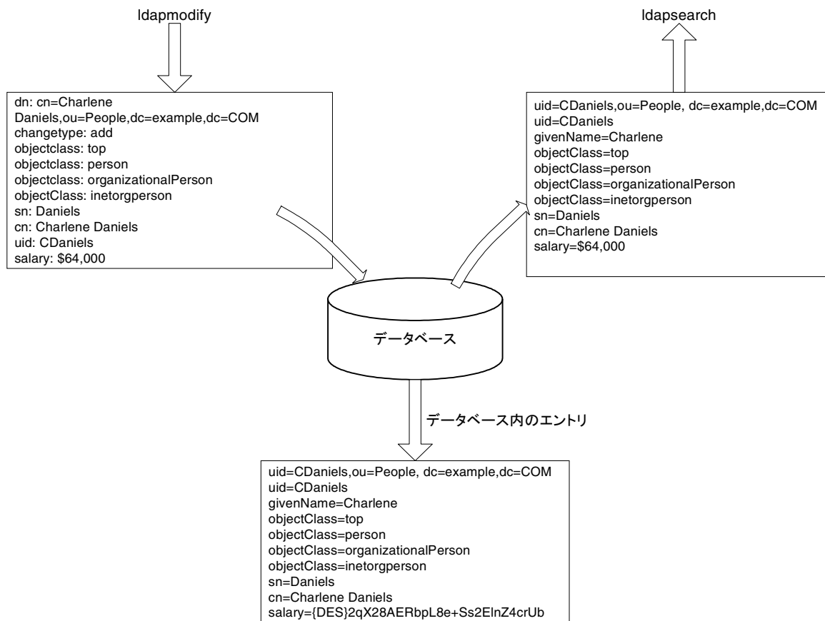
図 7-1 属性暗号化のロジック
