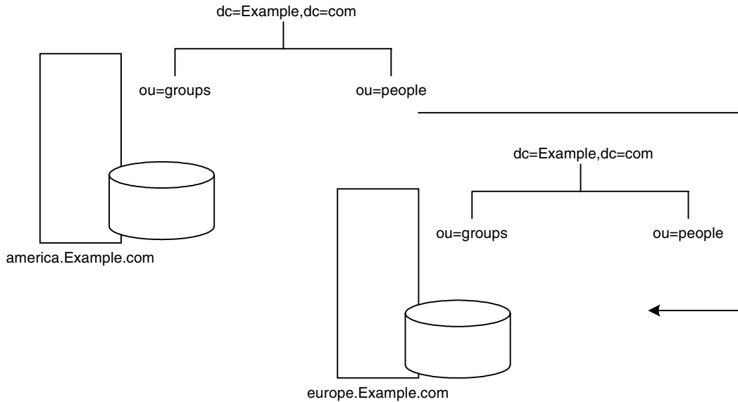
図 5-9 米国のディレクトリからヨーロッパのディレクトリへのスマートリフェラル
