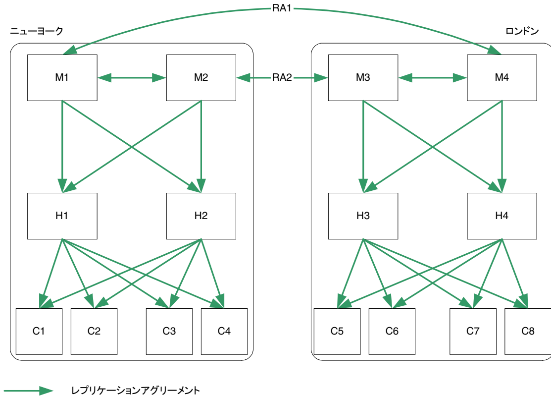
図 9-9 読み取りパフォーマンスのための2つのデータセンターのスケールアップ
