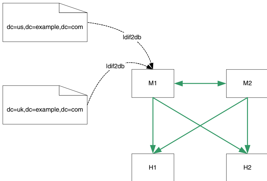
図 9-4 Idif2db による復元
