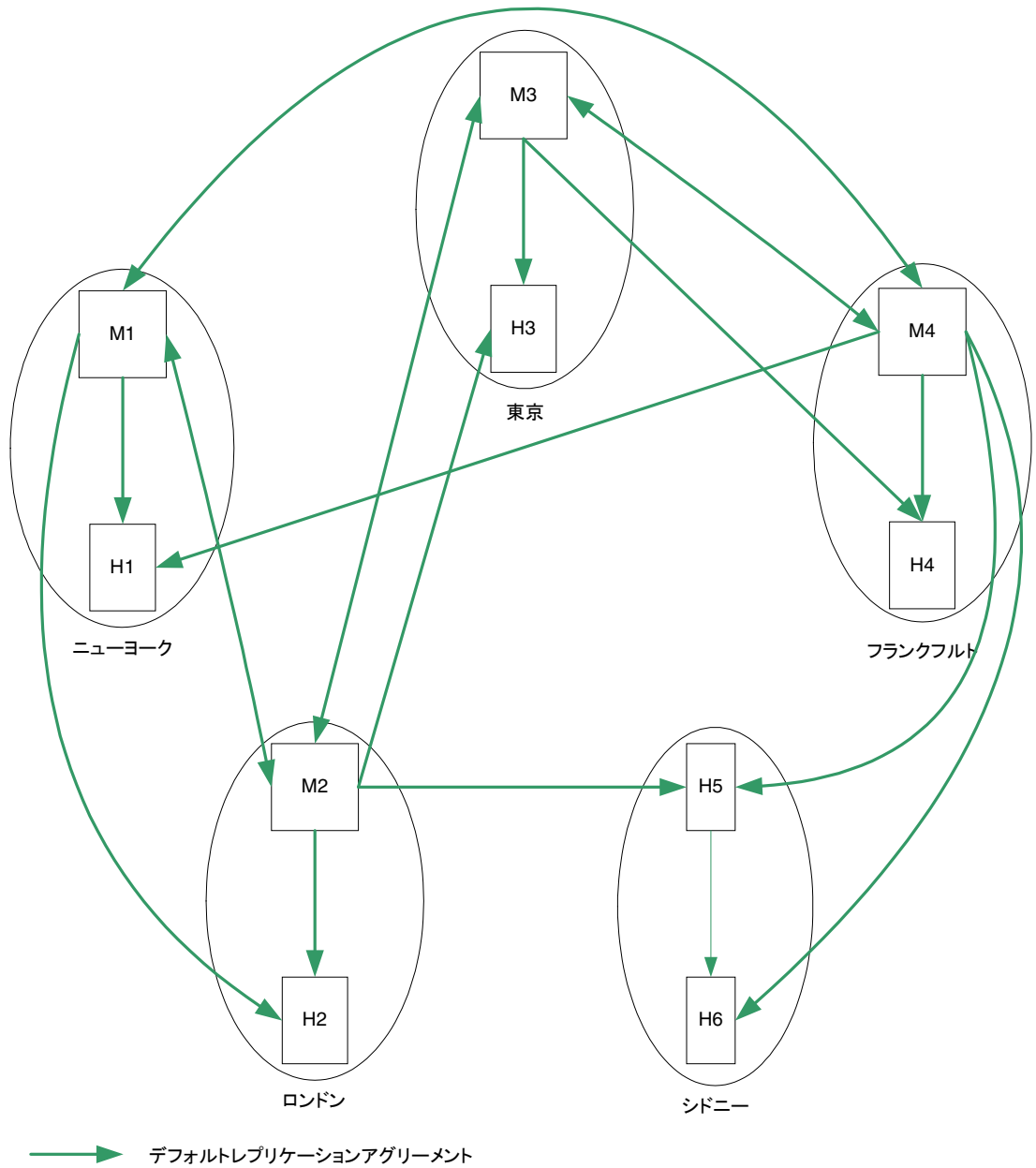
図 9-14 5つのデータセンターの基本トポロジ
