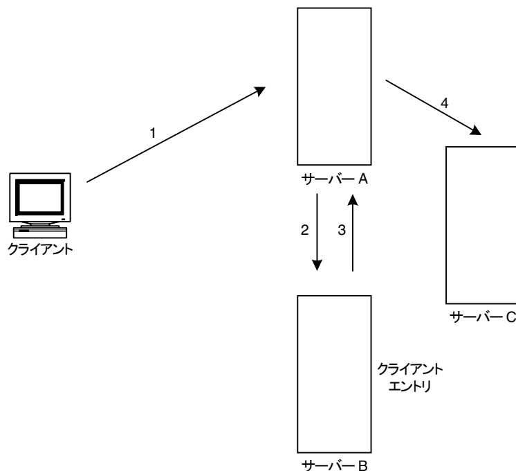
図 5-15 クライアントからの検索要求を処理するために2つの連鎖サフィックスを使用する連鎖
