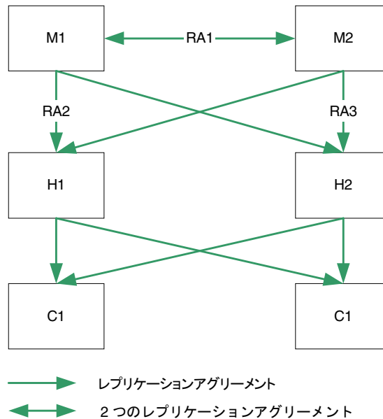
図 9-6 読み取りパフォーマンスのための1つのデータセンターのスケーリング
