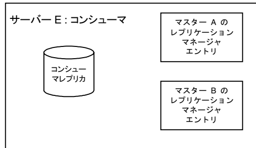
図 6-5 コンシューマサーバー E のレプリケーション設定 (完全にメッシュ化されたトポロジ)
