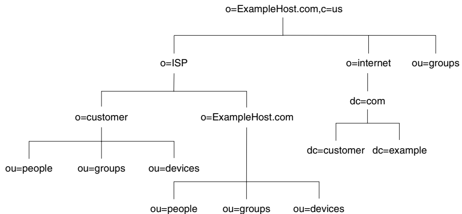
図 4-11 ExampleHost.com 社の詳細な DIT
