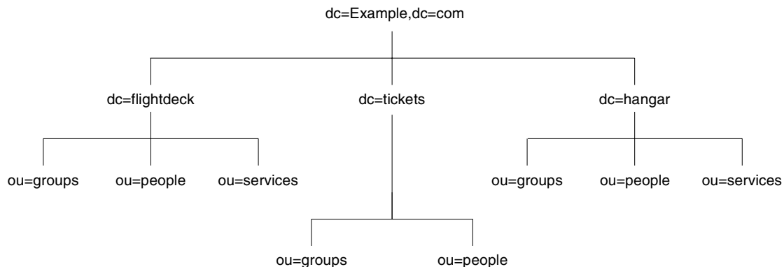
図 4-9 Example.com 社 DIT の 3 つの主要ネットワークの詳細
