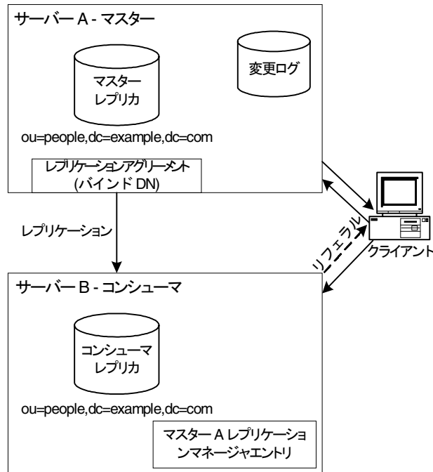
図 6-1 シングルマスターレプリケーション
