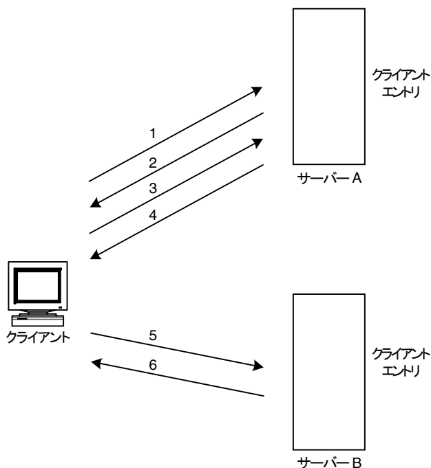
図 5-13 リフェラルによって転送されるクライアントアプリケーションの検索要求
