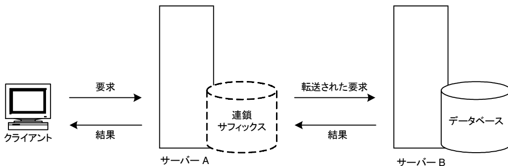
図 5-12 連鎖による処理
