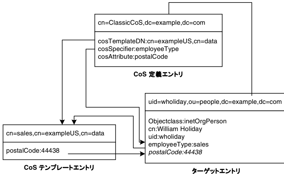
図 4-14 クラシック CoS の定義とテンプレートの例
