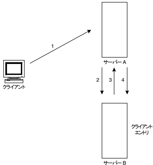
図 5-14 連鎖を使用した検索要求
