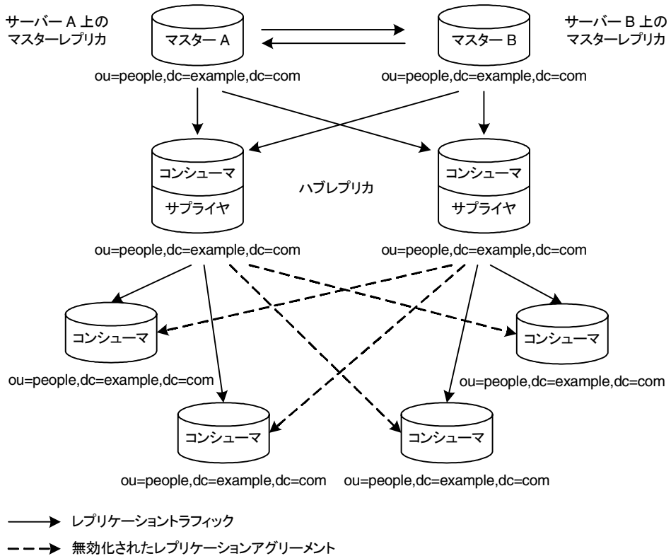
図 6-8 マルチマスターレプリケーションとカスケード型レプリケーションの組み合わせ
