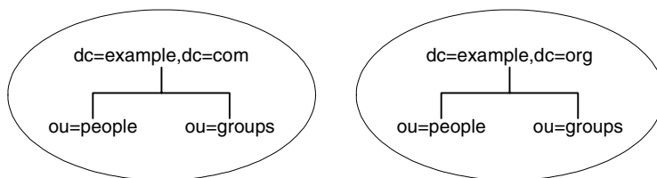
図 4-1 単一 Directory Server 内の2種類のルートサフィックス
