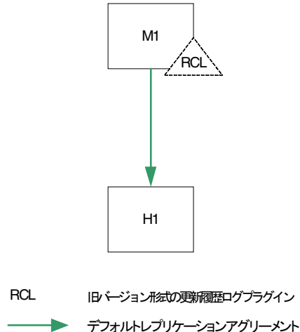
図 9-16 旧バージョン形式の更新履歴ログプラグインを使用する 1 つのデータセンター
