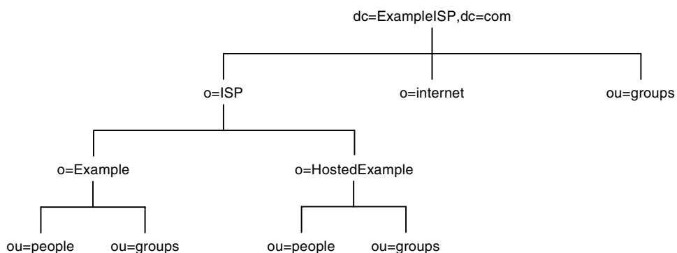
図 5-7 1つのサフィックスを持つ ExampleISP.com 社のディレクトリツリー
