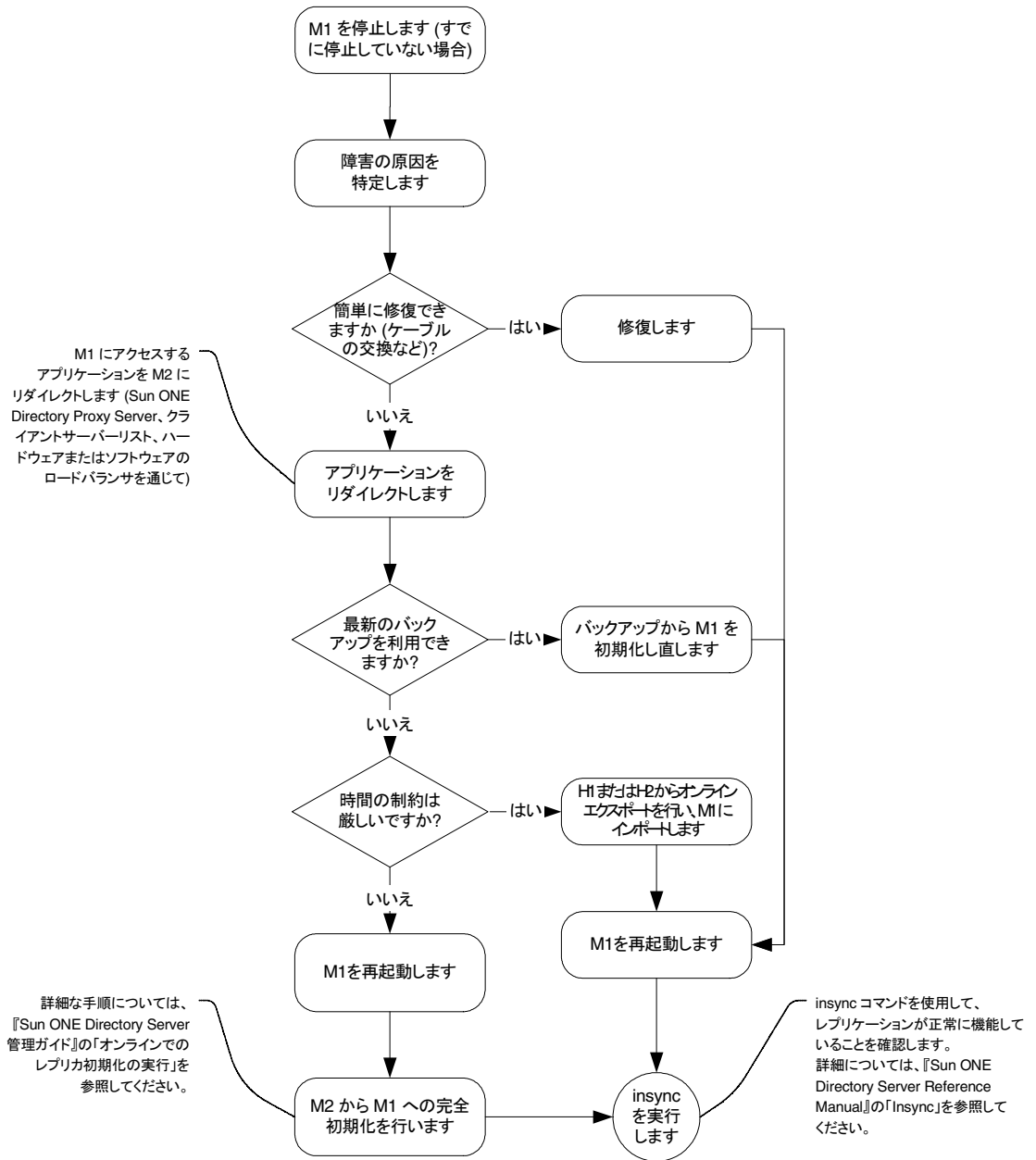
図 9-7 1つのデータセンターの復元手順を示すフローチャート(1つのコンポーネント)
