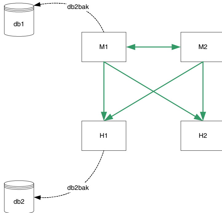
図 9-1 バイナリバックアップ
