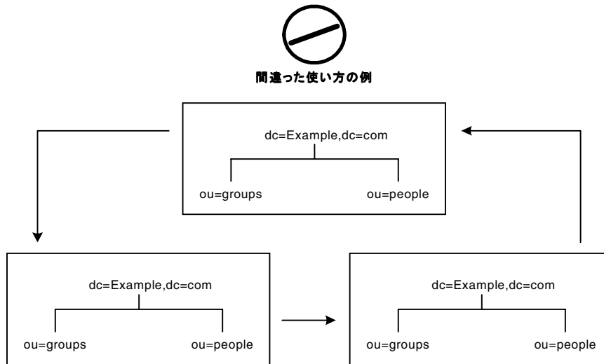
図 5-11 スマートリフェラルの使いすぎによる循環リフェラルのパターン
