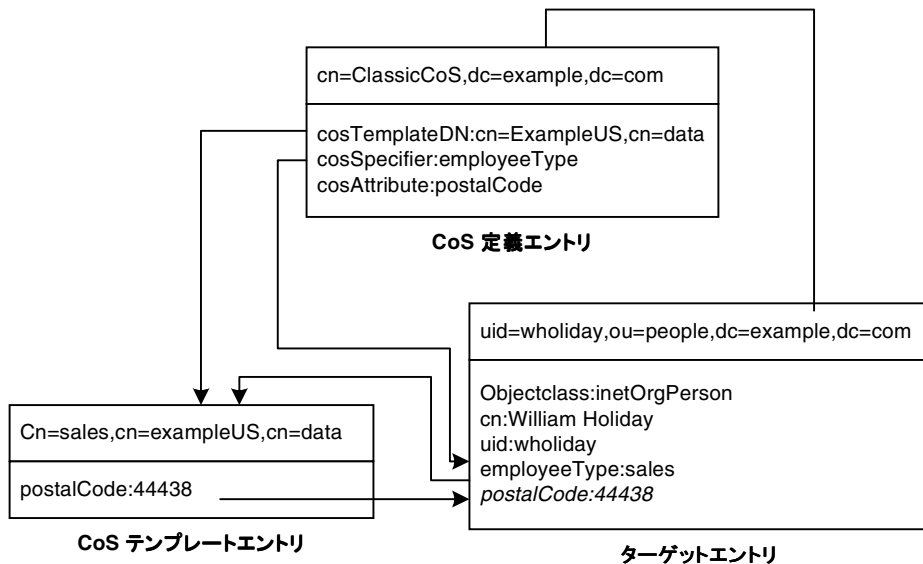
図 4-12 ポインタ CoS の定義とテンプレートの例
