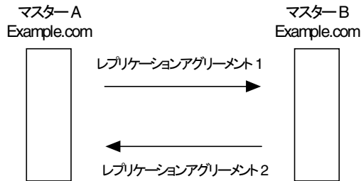
図 6-2 マルチマスターレプリケーションの設定 (2 つのマスター)
