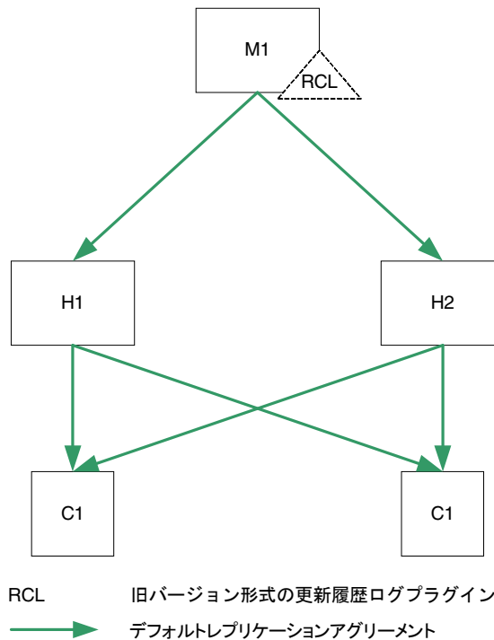
図 9-17 旧バージョン形式の更新履歴ログプラグインを使用する 1 つのデータセンター (スケーリング)
