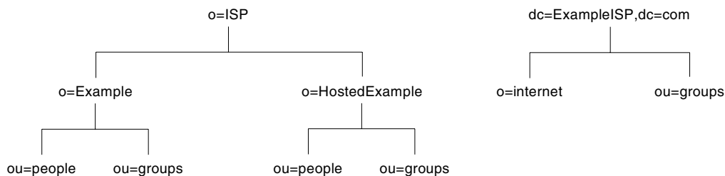
図 5-8 2つのサフィックスを持つ ExampleISP.com 社のディレクトリツリー
