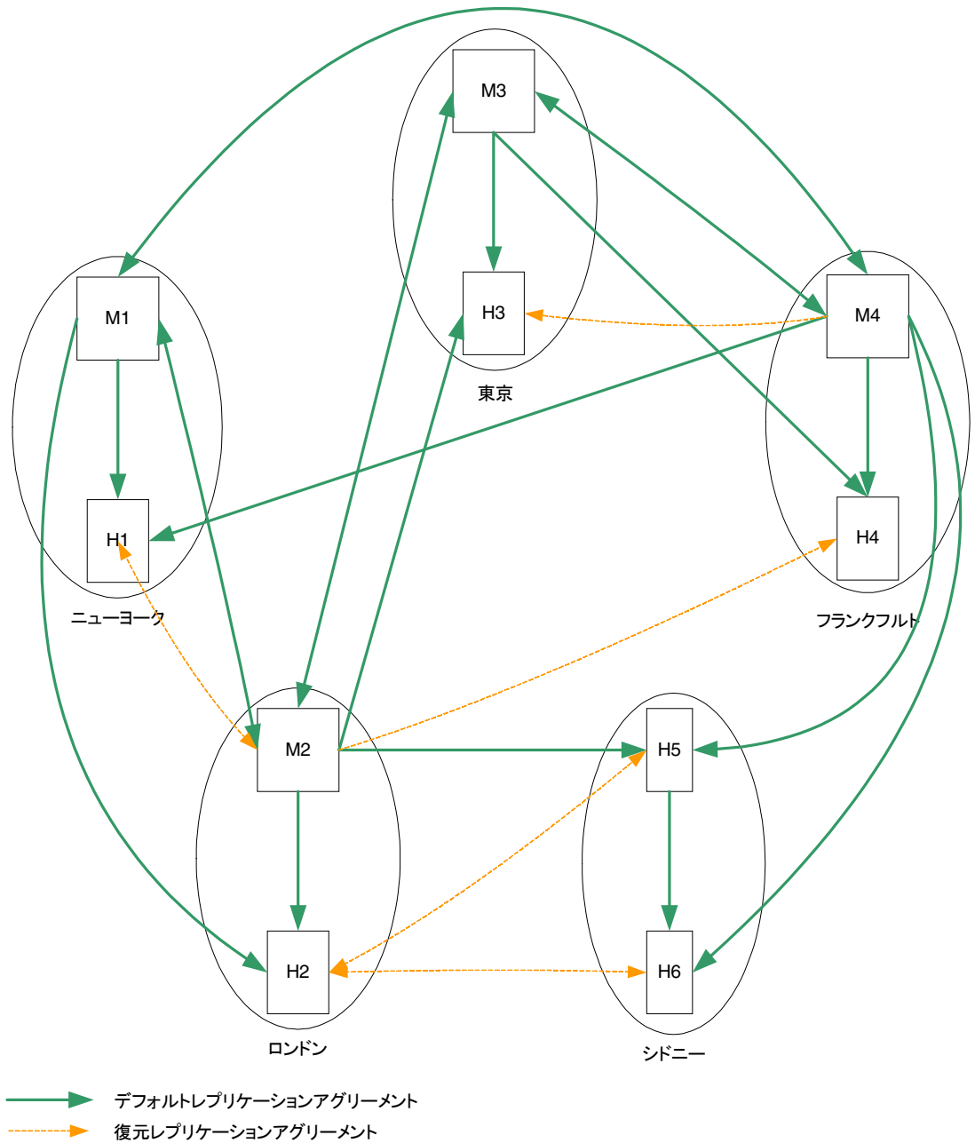
図 9-15 5つのデータセンターの復元レプリケーションアグリーメント
