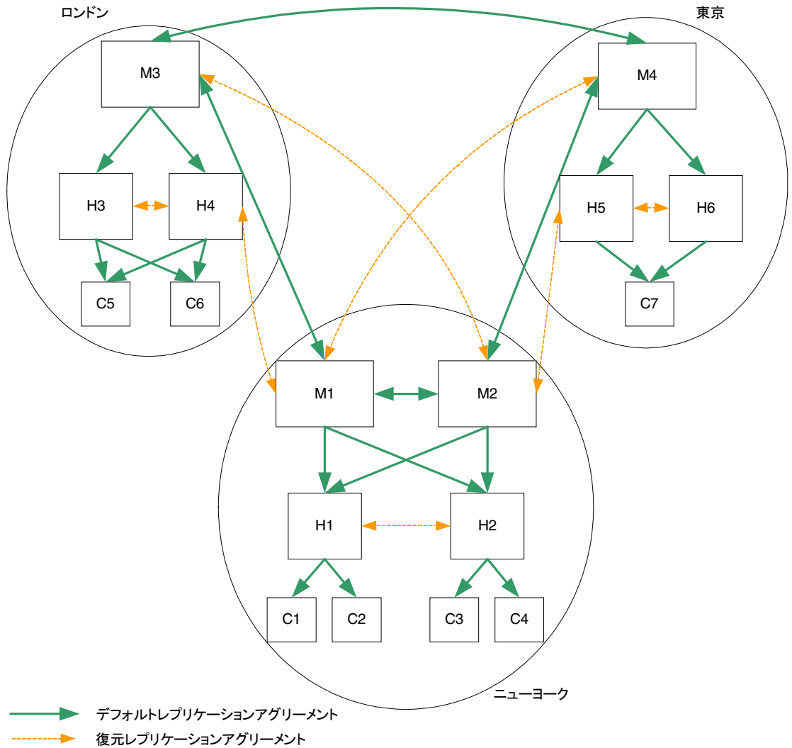
図 9-13 3つのデータセンターの復元レプリケーションアグリーメント
