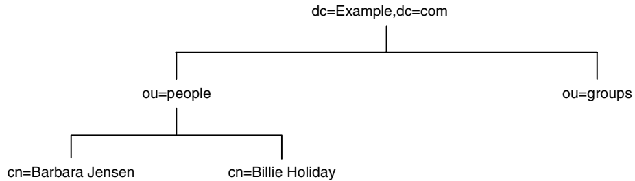
図 4-6 Example.com 社のディレクトリ情報ツリー
