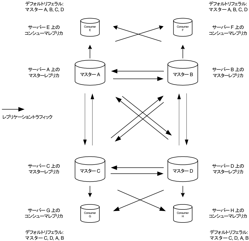
図 6-3 サフィックス「ou=people,dc=example,dc=com」の完全にメッシュ化された4方向のマルチマスターレプリケーション構成
