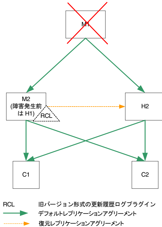
図 9-18 旧バージョン形式の更新履歴ログプラグインを使用する 1 つのデータセンター (復元)
