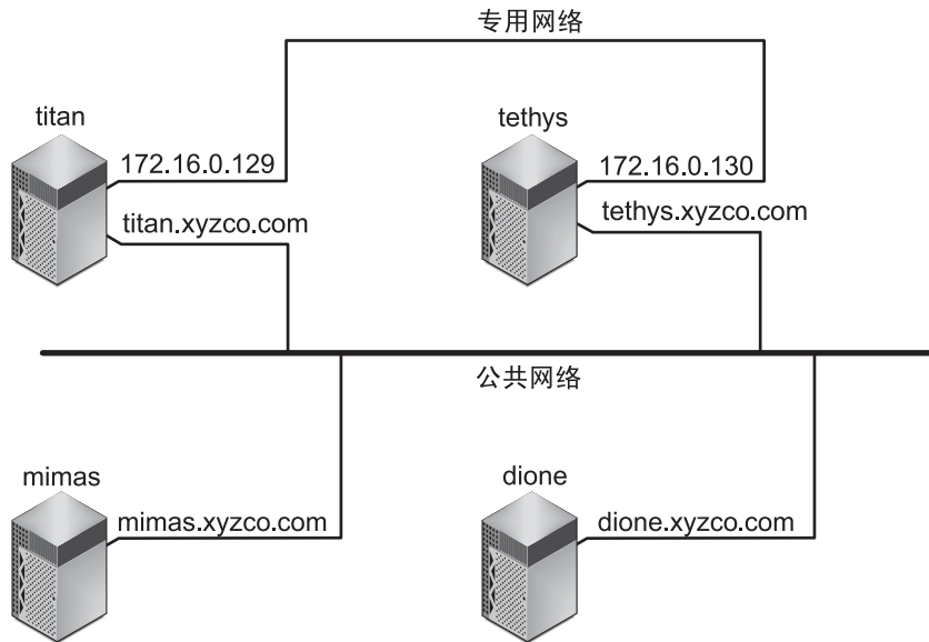
图 4-1 网络接口
