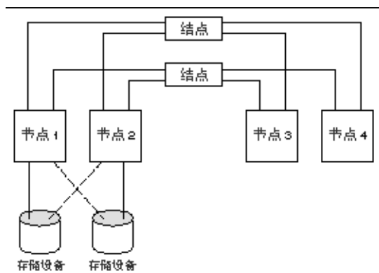
图 2-3 SPARC: Pair+N 拓扑
