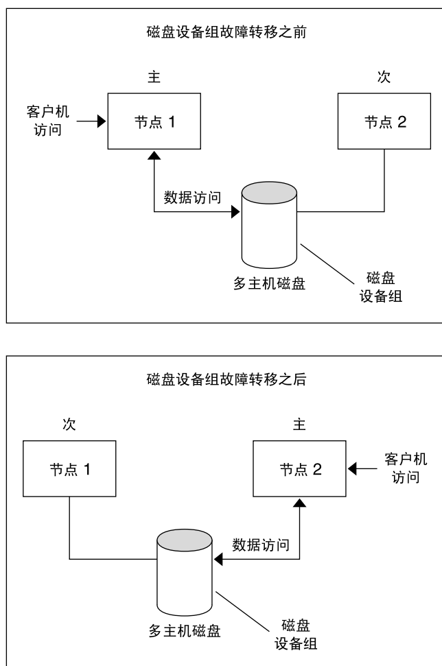
图 3-1 磁盘设备组失效转移
