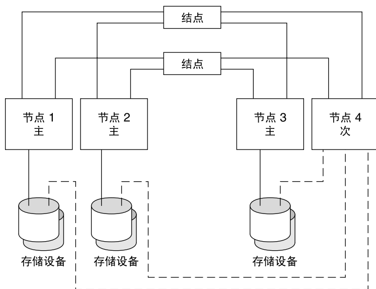
图 2-4 SPARC: N+1 拓扑
