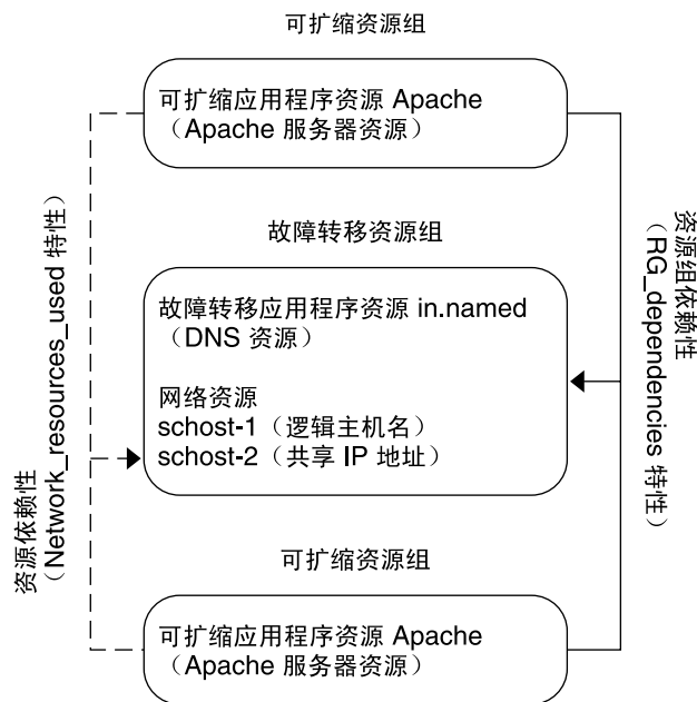
图 3-7 SPARC: 失效转移和可伸缩资源组示例
