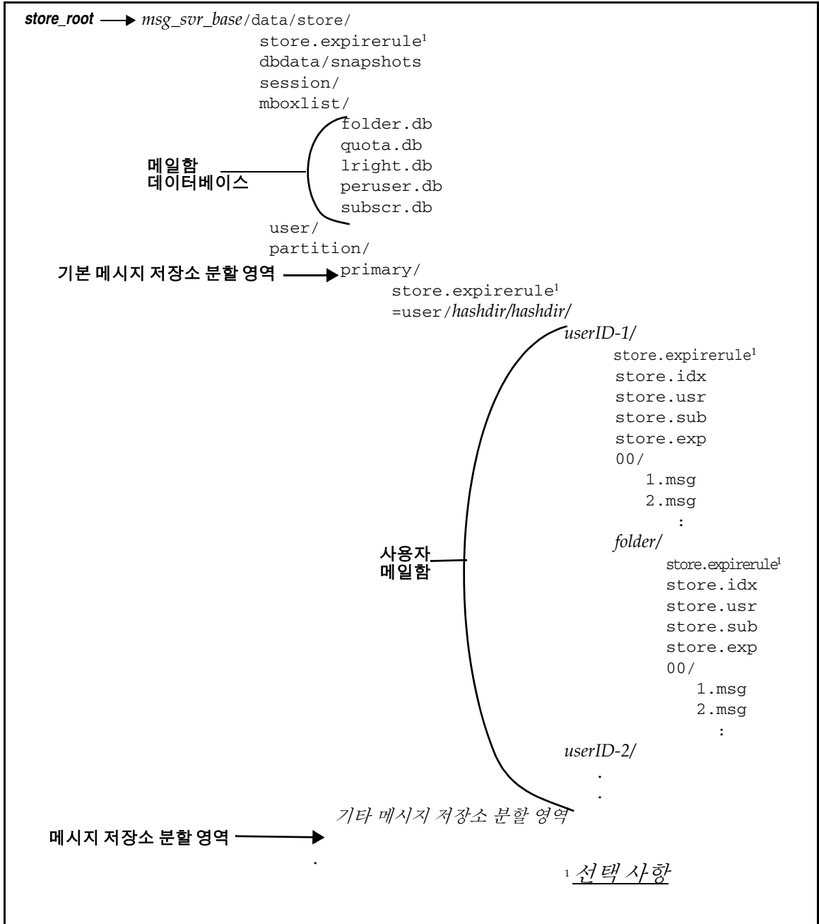
그림 18-1 메시지 저장소 디렉토리 레이아웃
