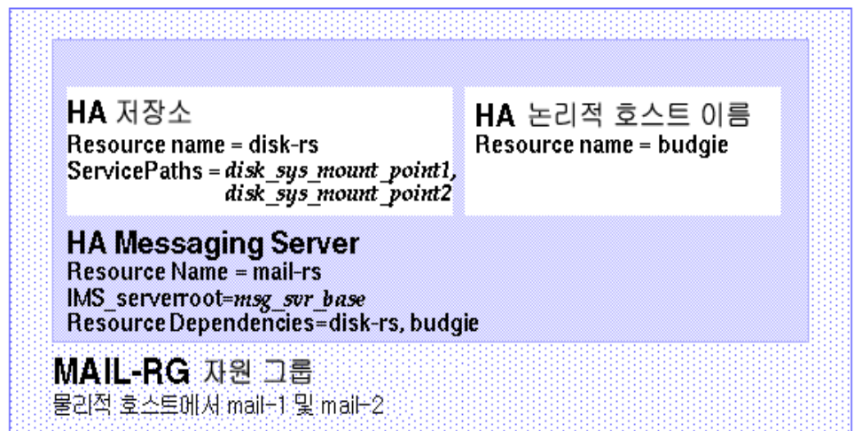
그림 3-3 간단한 Sun Java System Messaging Server HA 구성
