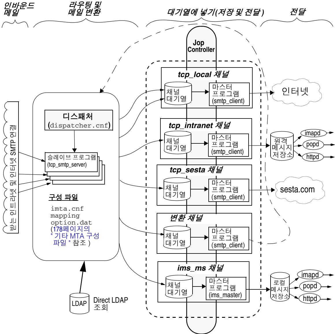
그림 8-2 MTA 구조
