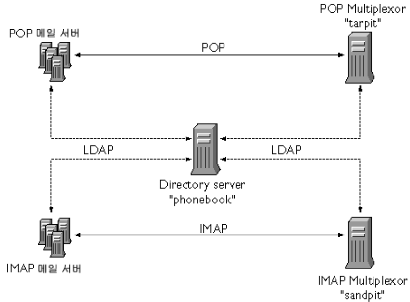
그림 7-2 여러 Messaging Server를 지원하는 여러 MMP
