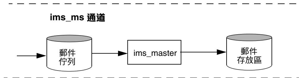
圖 8-4 ims-ms 通道
