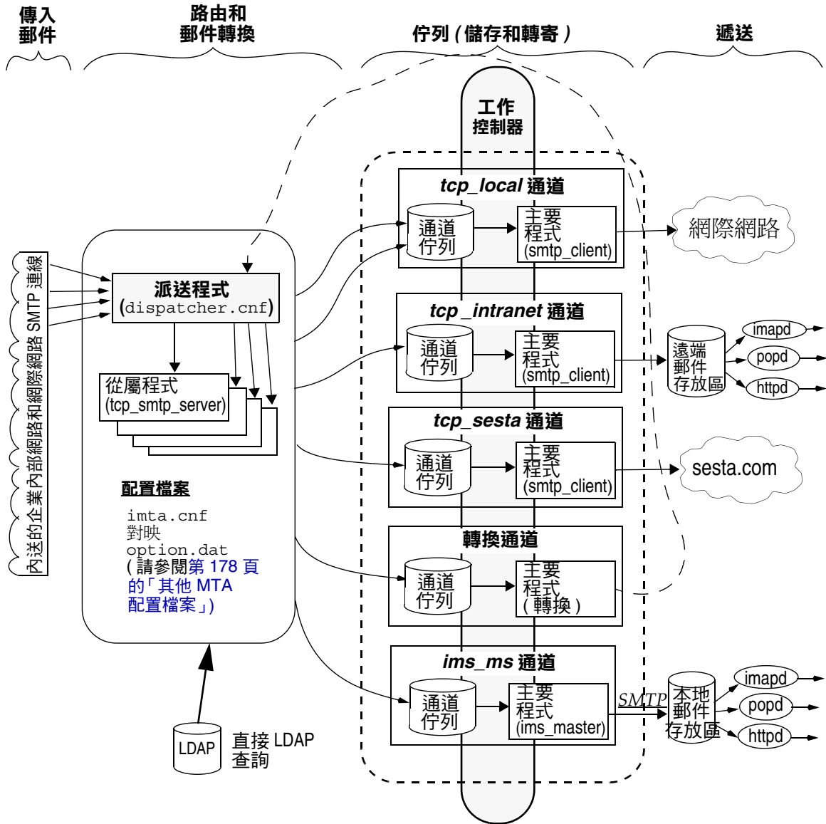
圖 8-2 MTA 架構
