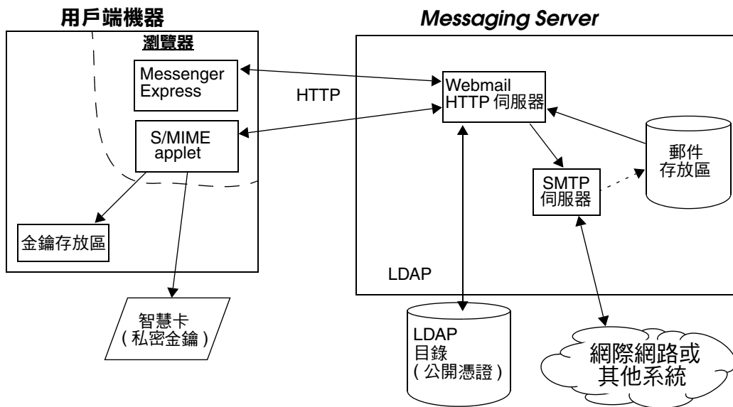
圖 20-1 S/MIME applet
