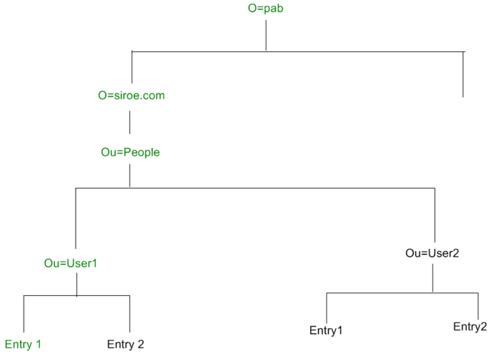
図 7-2 PAB ツリーでの Entry1 の場所
