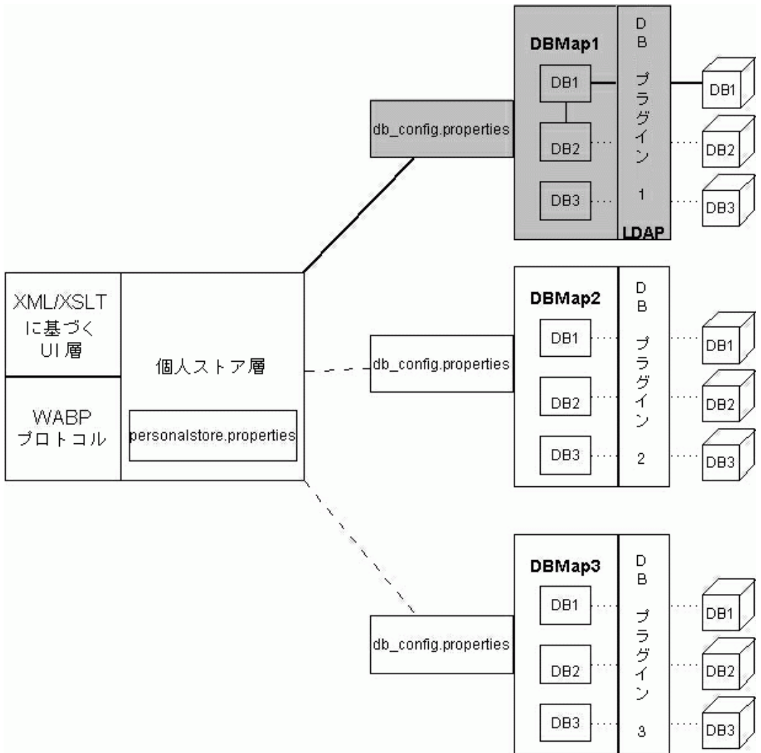
図 3-1 アドレス帳の水平方向のスケールビリティ
