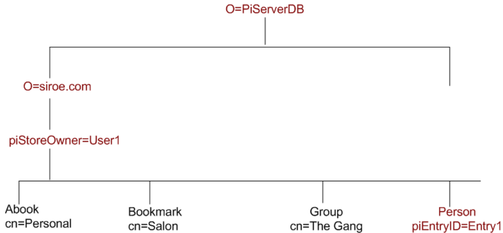
図 7-3 アドレス帳サーバーツリー内の Entry1 の場所
