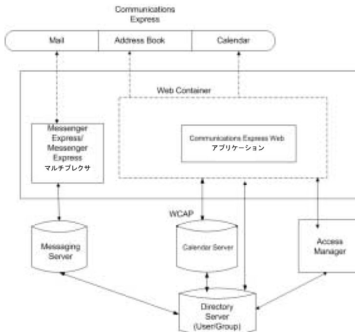
図 1-1 高レベルのアーキテクチャ
