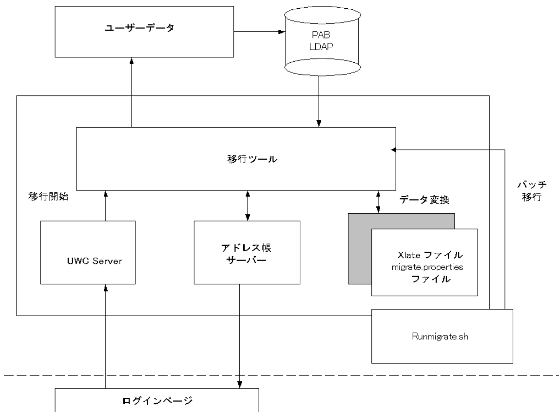
図 7-1 データ移行プロセスの概要
