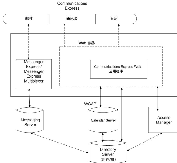
图 1-1 高级体系结构
