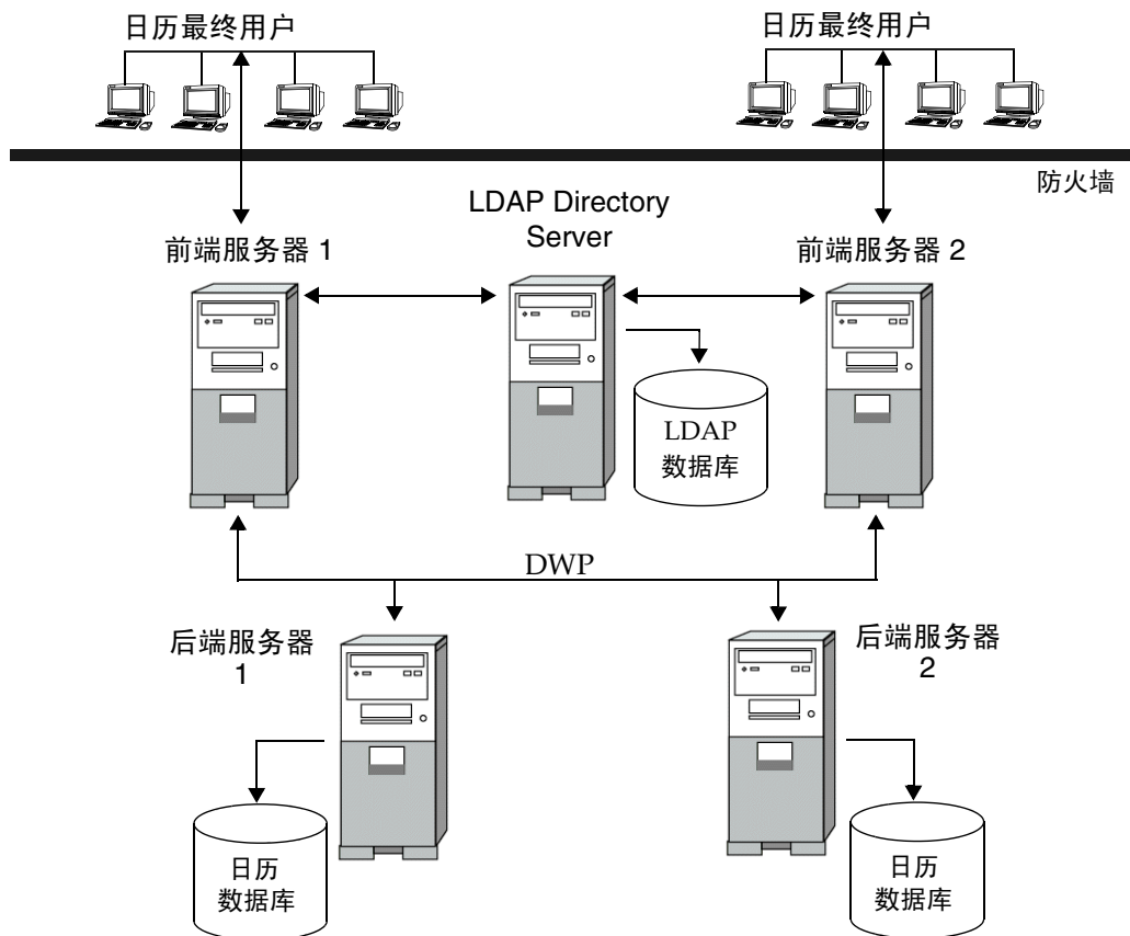
图 6-1 多个前端服务器与多个后端服务器
