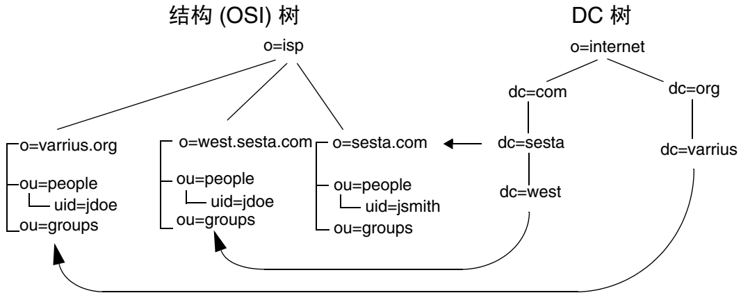
图 11-2 使用 LDAP Schema 1 的 LDAP 目录结构
