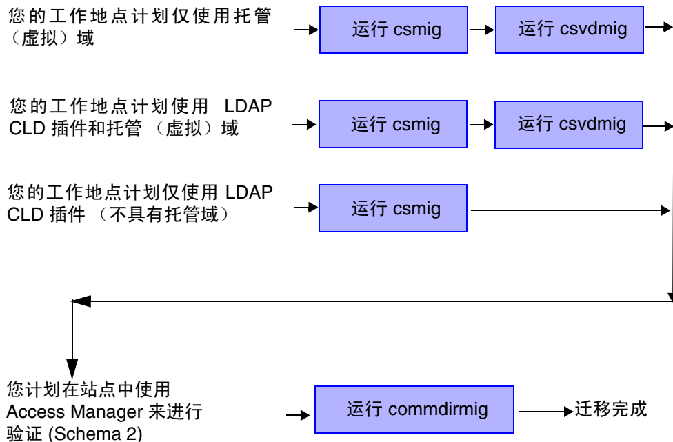
图 4-1 选择要运行的迁移实用程序
