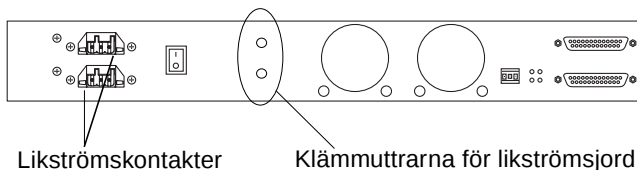
BILD 3-22 Ansluta likströmsjordkabeln
