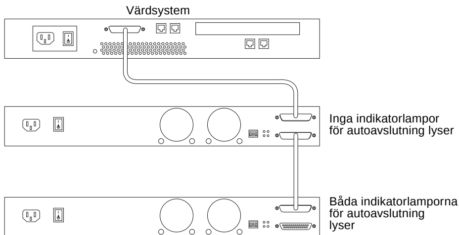
BILD 5-5 Indikatorlampor för autoavslutning i en Ultra-SCSI eller Wide-SCSI-kedja
