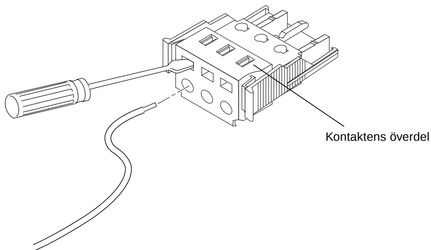
BILD 2-7 Öppna likströmskontaktens fjäderklämma med en skruvmejsel
