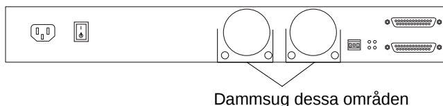
BILD 5-13 Rengöra fläktarna på baksidan
