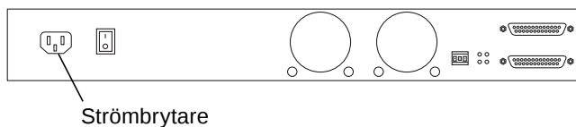
BILD 3-21 Ansluta växelströmskabeln
