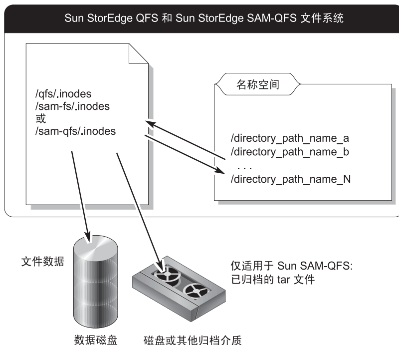
图 4-1 Sun StorEdge QFS 文件系统中的 .inodes 文件
