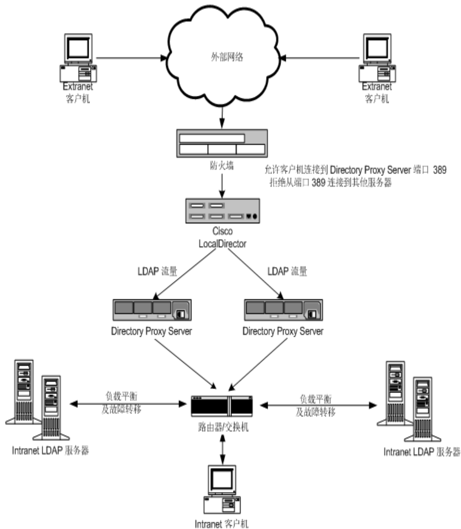
图 2-4 Directory Proxy Server 使用单防火墙的设置
