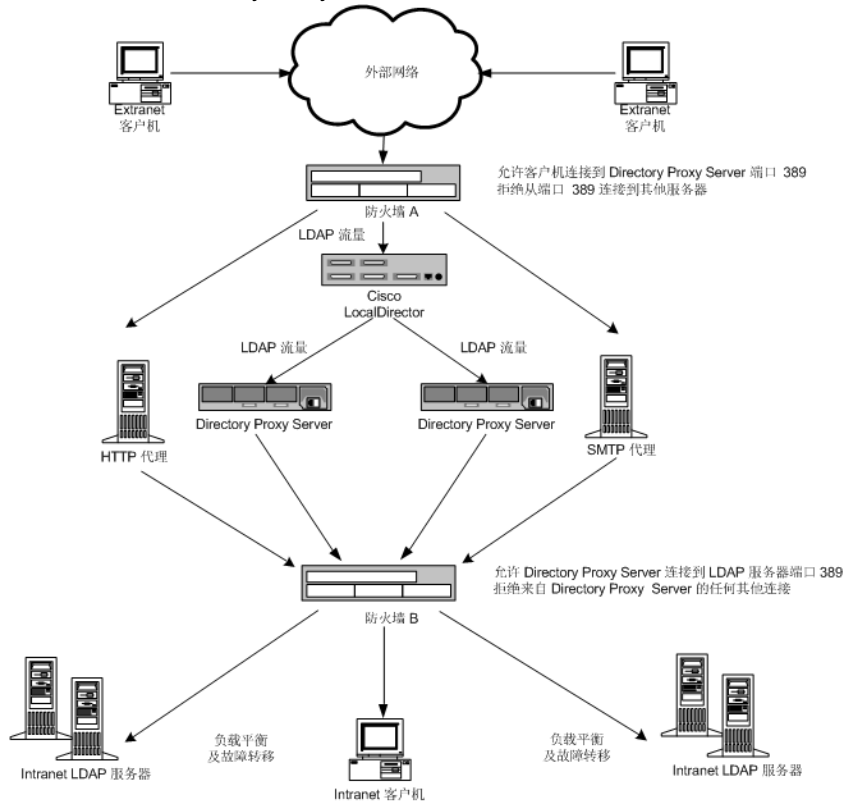
图 2-5 Directory Proxy Server 使用双防火墙的设置
