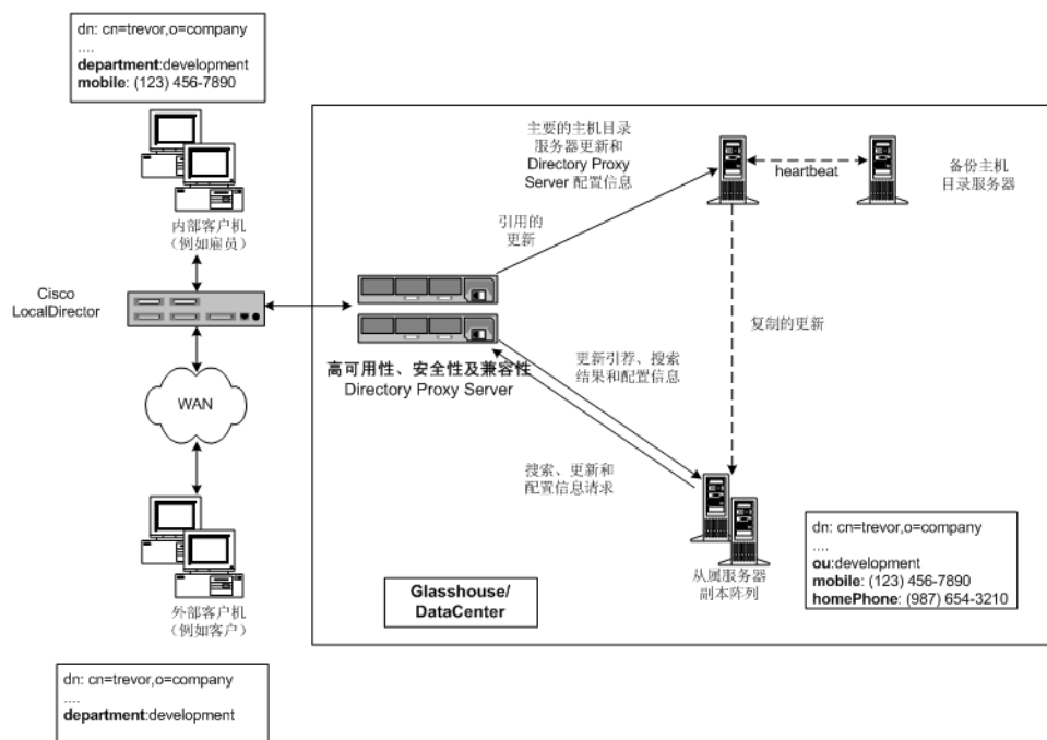
图 2-3 集中式 LDAP 目录架构
