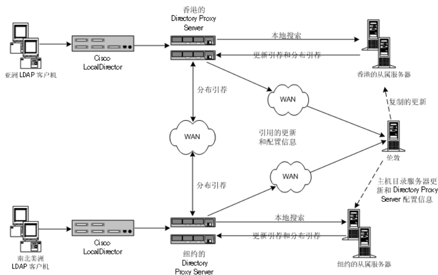
图 2-2 分布式 LDAP 目录架构
