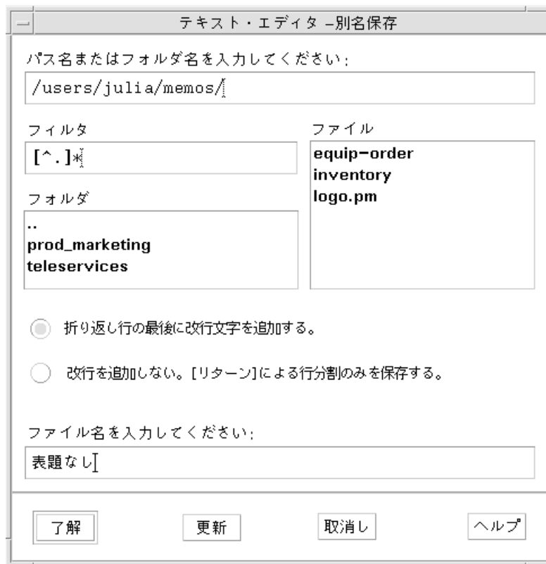
図 10-2 [別名保存] ダイアログ・ボックス
