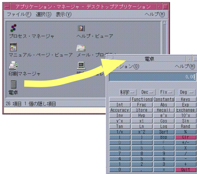
図 6-4 アプリケーション・マネージャからアプリケーションのウィンドウを開く
