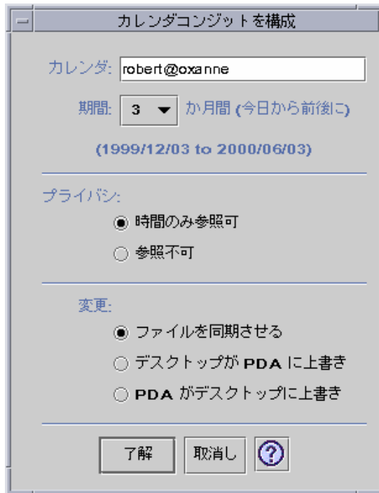
図 20-4 カレンダー・コンジットの構成
