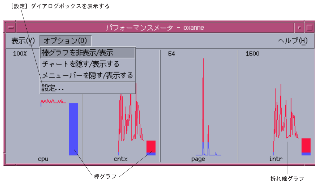
図 18-1 パフォーマンスメータですべてのパラメータを折れ線グラフで (横に) 表示する
